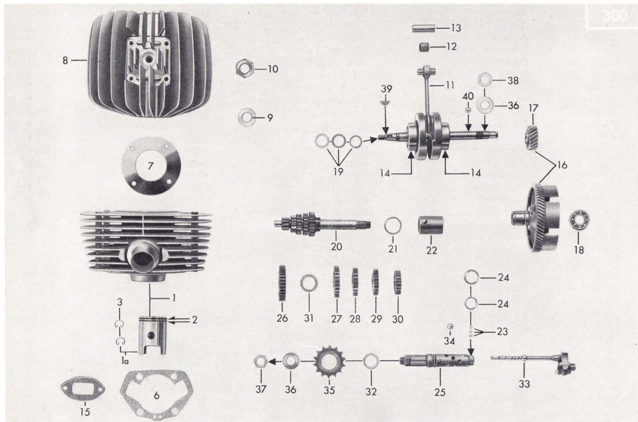
Tafel 4/1 Zylinder, Kurbelwelle, Getriebe Table 4/1 Cylinder, crankshaft, gearbox Planche 4/1 Cylindre, vilebrequin, boîte de vitesses
