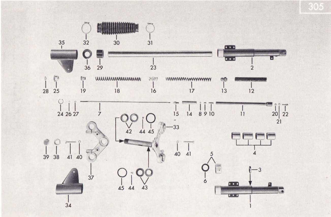
Tafel 10/1 Teleskopgabel, Lenkungslager Table 10/1 Telescopic fork, handlebar bearing Planche 10/1 Fourche télescopique, palier de direction
