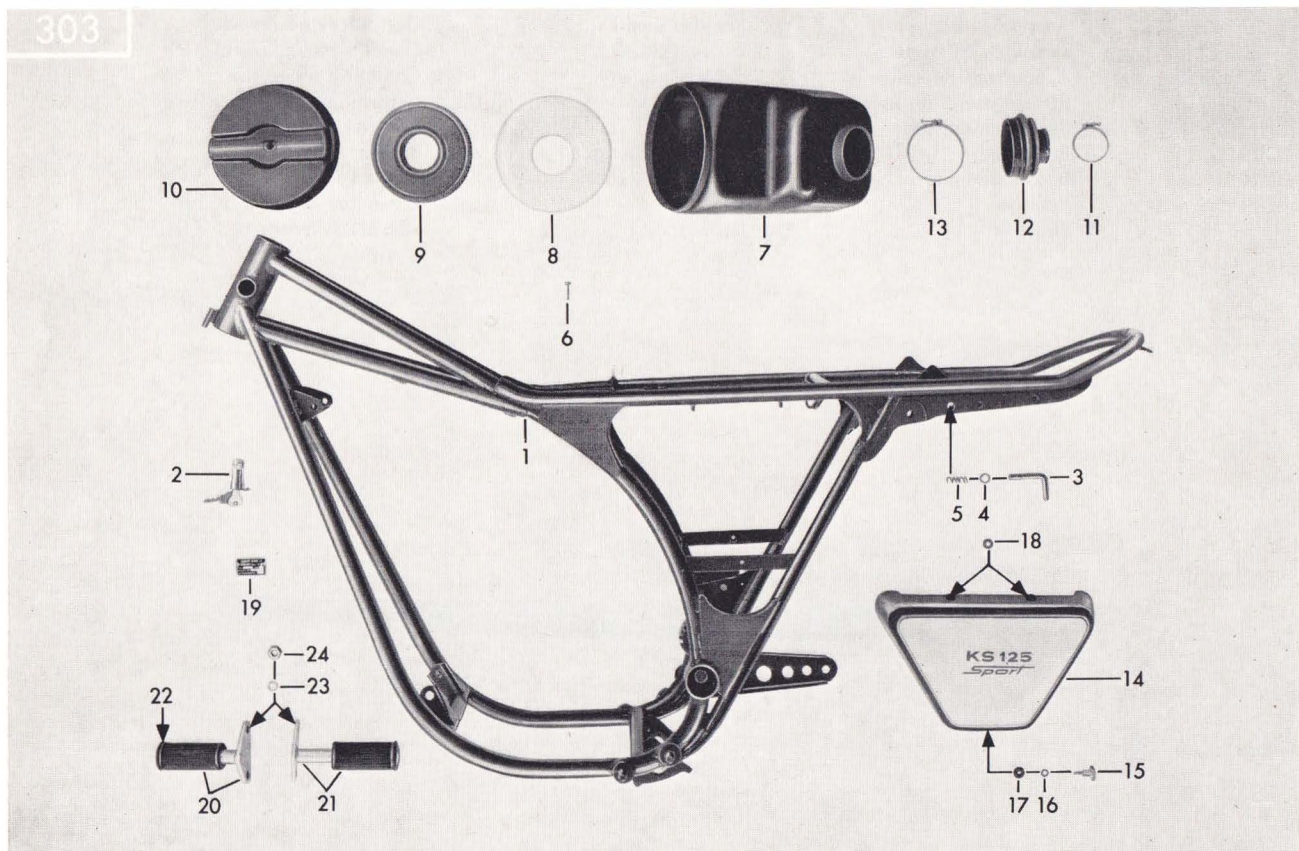
Tafel 8/1 Rahmen, Rahmendeckel, Geräuschdämpfer, Fußrasten Table 8/1 Frame, frame cover, noise damper, foot rests Planche 8/1 Cadre, couvercle de cadre, amortisseur de bruit, repose-pieds
