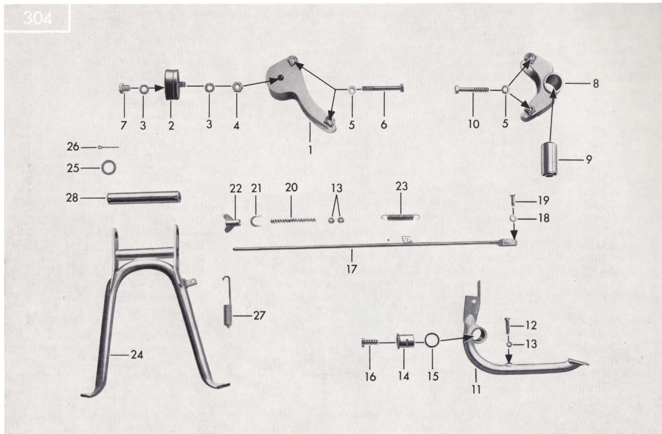
Tafel 9/1 Motoraufhängung, Fußbremse, Radständer Table 9/1 Engine mounting, foot brake, centre prop Planche 9/1 Suspension de moteur, frein à pied, béquille
