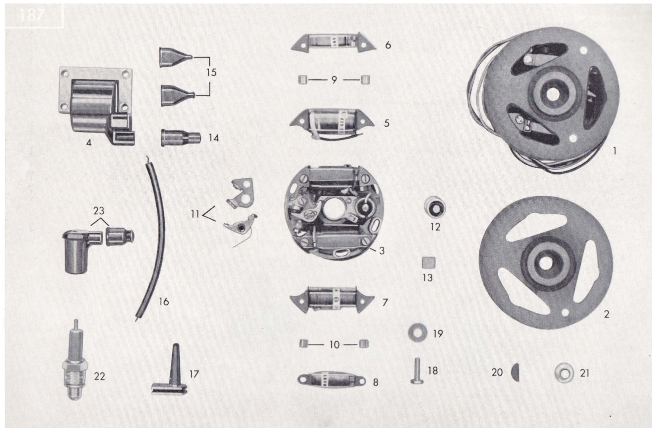
Tafel 6/1 Schwunglicht-Magnetzünder Table 6/1 Flywheel magneto Planche 6/1 Volant magnétique
