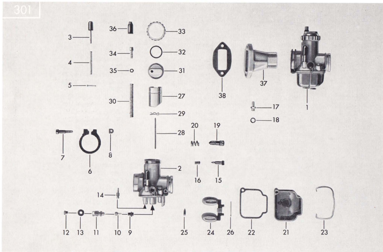
Tafel 5/2 Vergaser, Ansaugstutzen Table 5/2 Carburettor, suction socket Planche 5/2 Carburateur, tubulure d'aspiration
