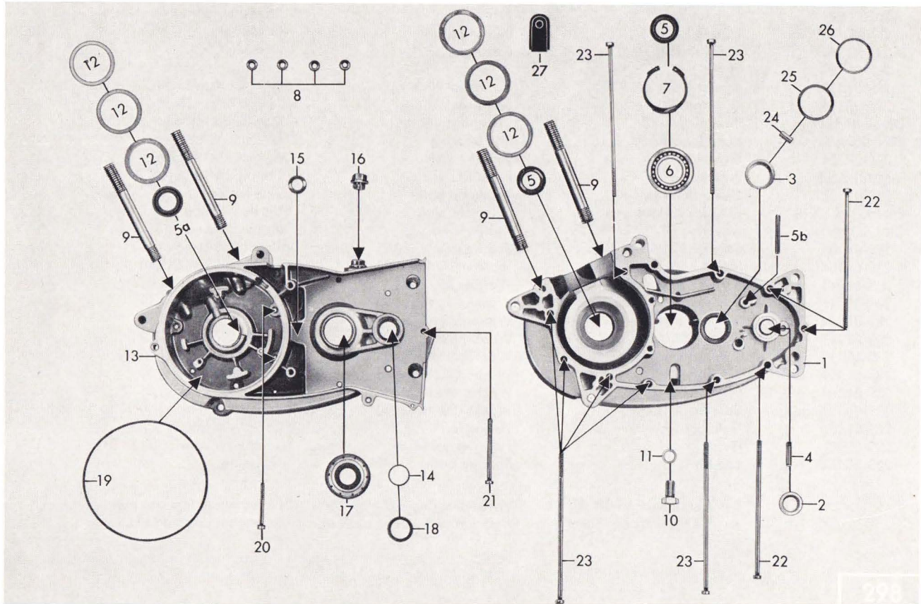
Tafel 1/2 Gehäuse rechts, Gehäuse links Table 1/2 Casing right, casing left Planche 1/2 Carter droite, carter gauche
