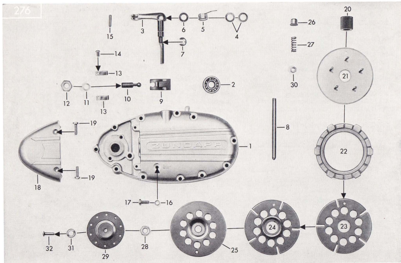
Tafel 3/1 Gehäusedeckel rechts, Kupplung Table 3/1 Casing cover right, clutch Planche 3/1 Couvercle de carter droite, embrayage
