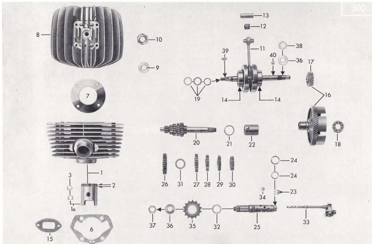
Tafel 4/2 Zylinder, Kurbelwelle, Getriebe Table 4/2 Cylinder, crankshaft, gearbox Planche 4/2 Cylindre, vilebrequin, boîte de vitesses
