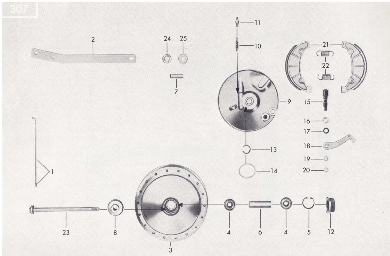
Tafel 12/1 Vorderrad, Nabe Table 12/1 Front wheel, front wheel hub Planche 12/1 Roue AV, moyeu de roue AV
