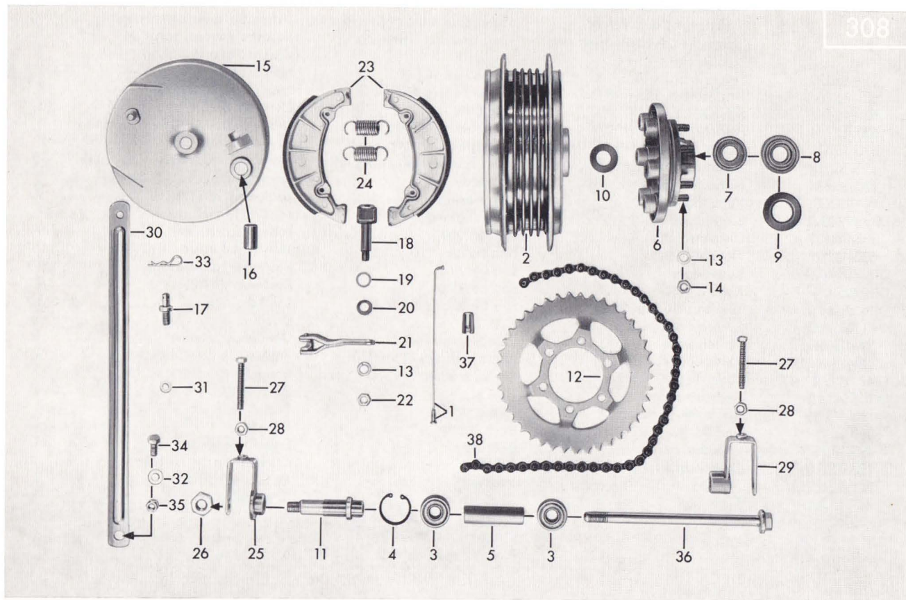
Tafel 13/2 Hinterrad, Nabe, Kettenrad, Kette Table 13/2 Rear wheel, rear wheel hub, chain sprocket, chain Planche 13/2 Roue AR, moyeu de roue AR, roue à chaîne, chaîne
