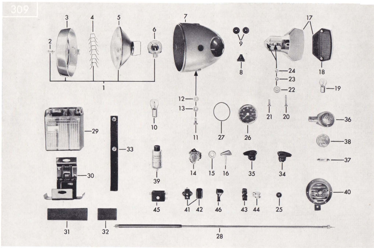
Tafel 14/1 Elektrische Ausrüstung Table 14/1 Electrical equipment Planche 14/1 Equipement électrique
