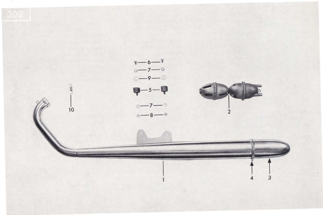
Tafel 7/1 Auspuffanlage Table 7/1 Exhaust system Planche 7/1 Système d'échappement
