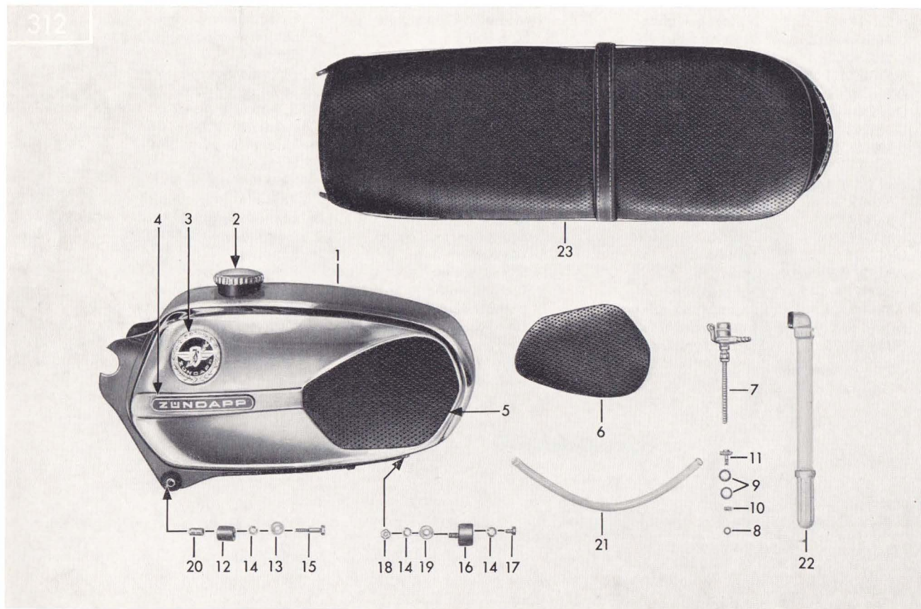
Tafel 17/1 Tank, Sitzbank, Werkzeug-Satz, Luftpumpe Table 17/1 Fuel tank, bench seat, tool set, air pump Planche 17/1 Réservoir, siège, outillage, pompe à air
