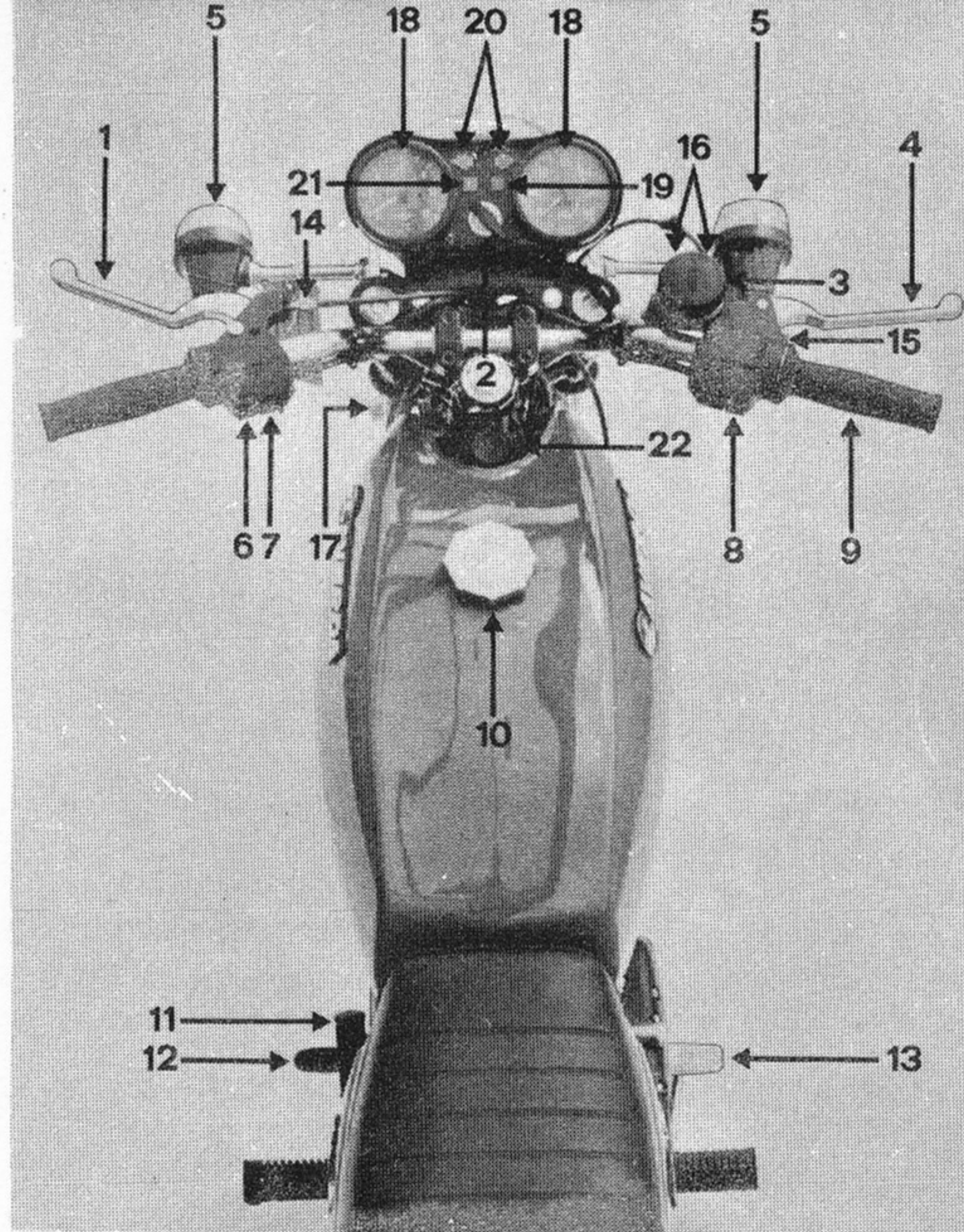
Fig. 1 - Disposizione comandi
