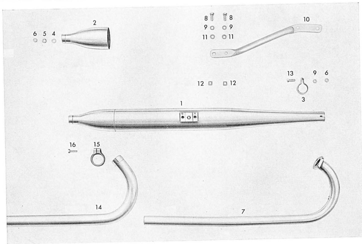
Tafel 12 c Auspuff (Inland)
