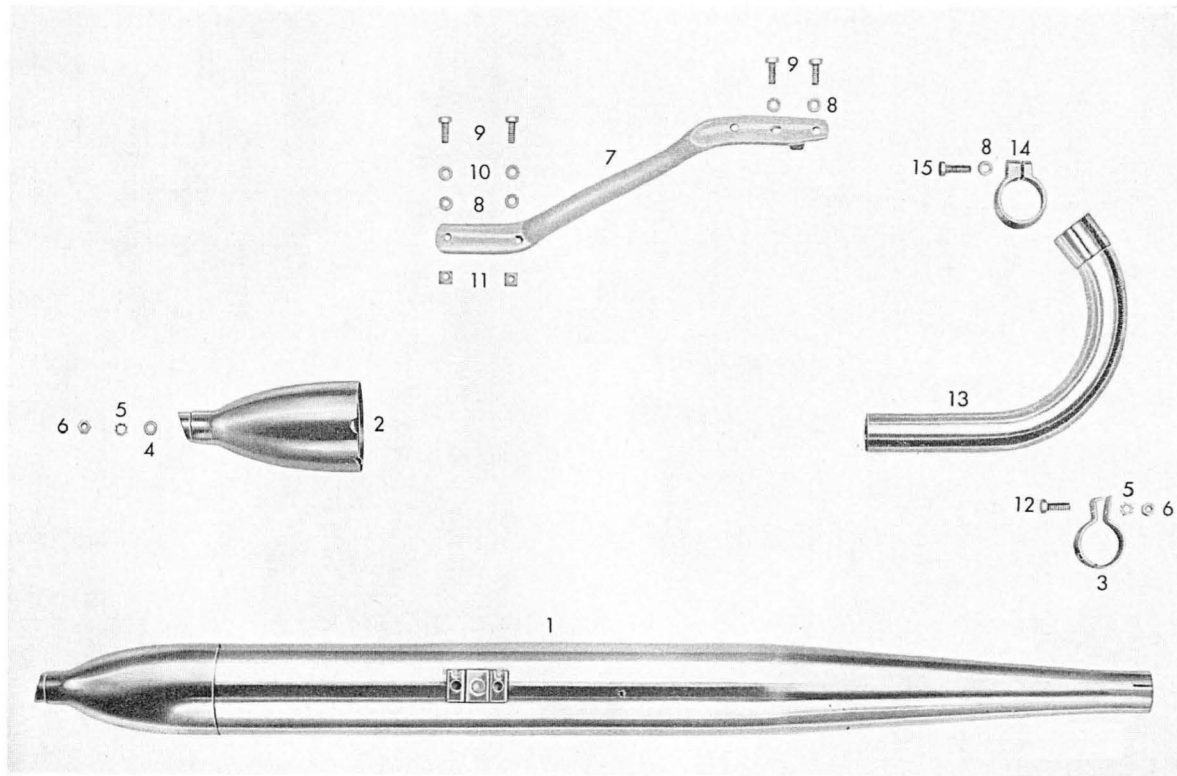
Tafel 12/1 Auspuff (Export)
