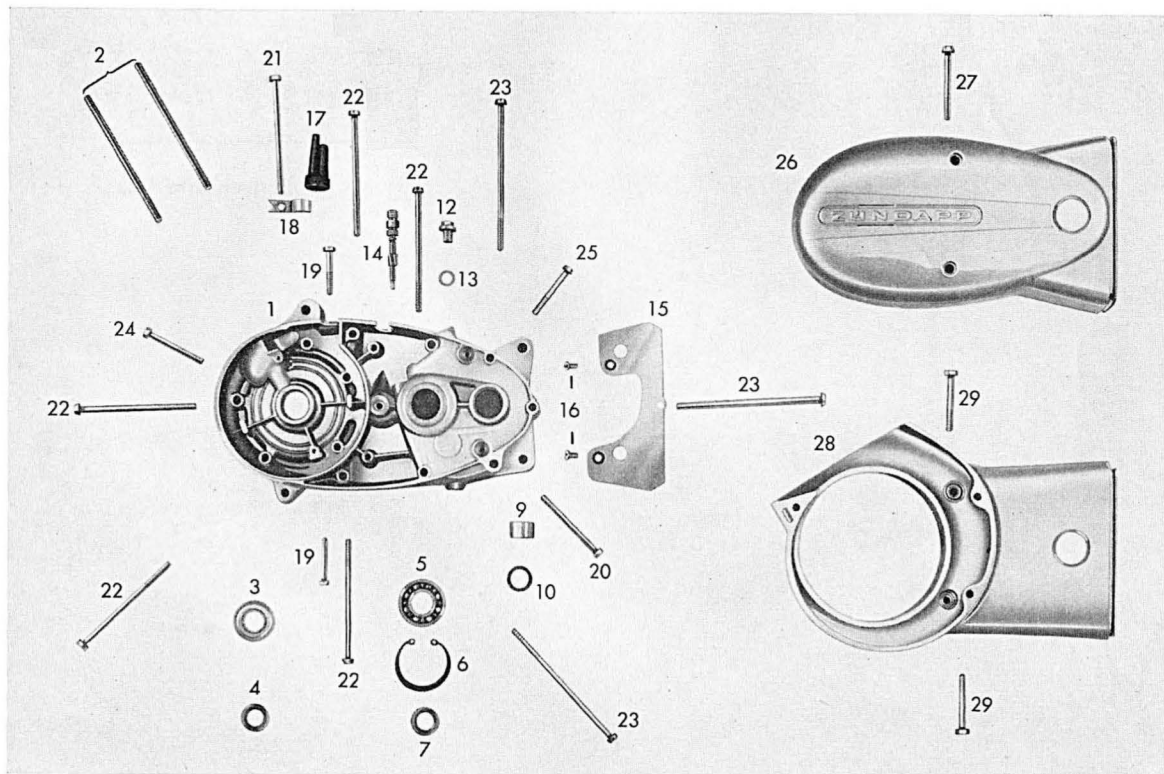
Tafel 2 b Gehäusehälfte links
