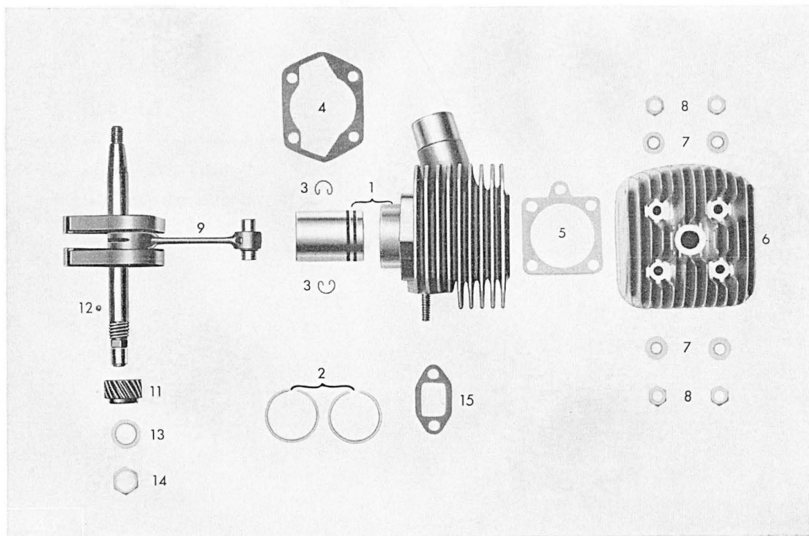
Tafel 5 c/1 Zylinder – Kurbeltrieb (nur für Motoren mit Gebläse)
