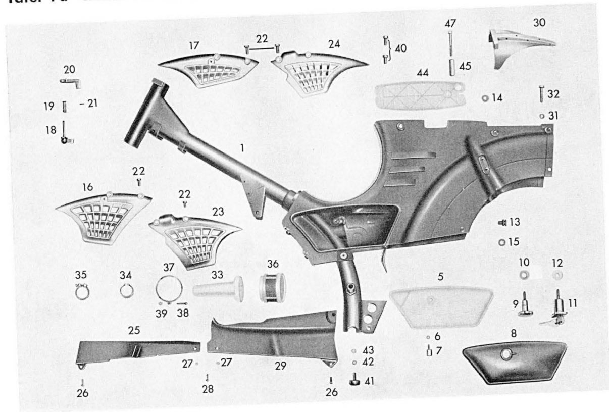
Tafel 1 a Rahmen - Mittelteil
