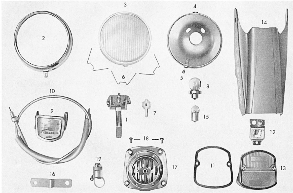
Tafel 7 a Lichtanlage - Tachometer - Rücklicht (dauerabgeblendet)
