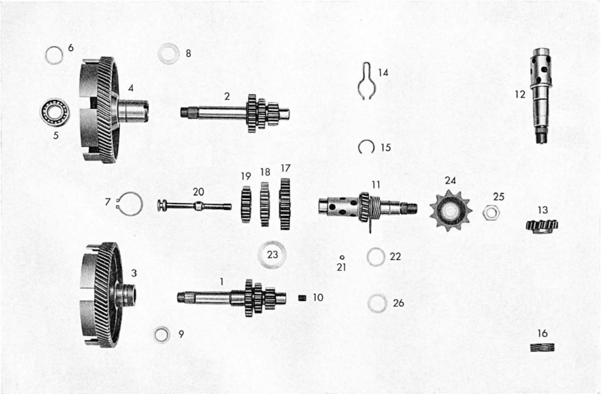
Tafel 7 Getriebe-Schaltwelle
