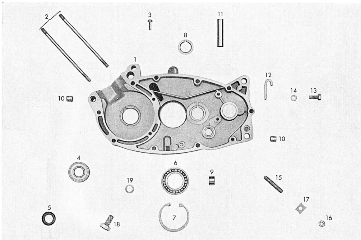
Tafel 1 Gehäusehälfte rechts
