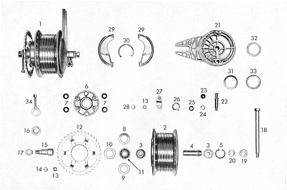
Tafel 6 Hinteres Laufrad - Hinterradnabe
