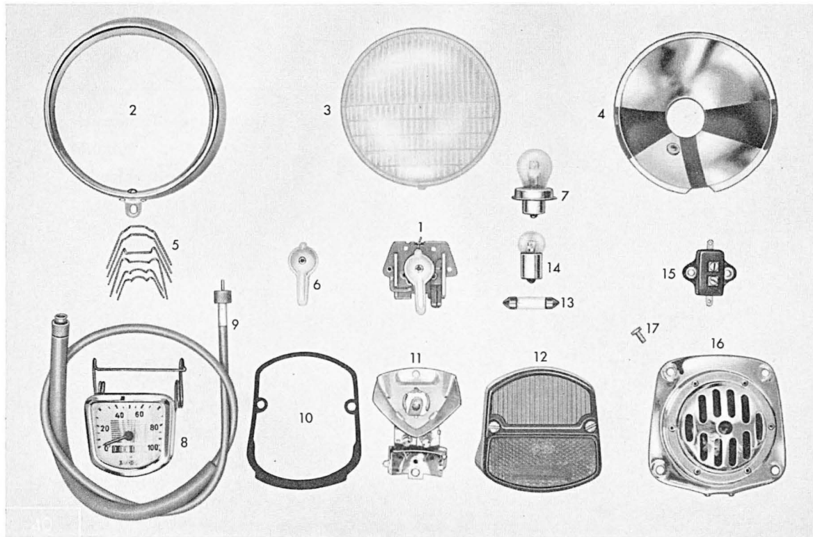
Tafel 7 b Lichtanlage – Tachometer – Rücklicht (dauerabgeblendet)
