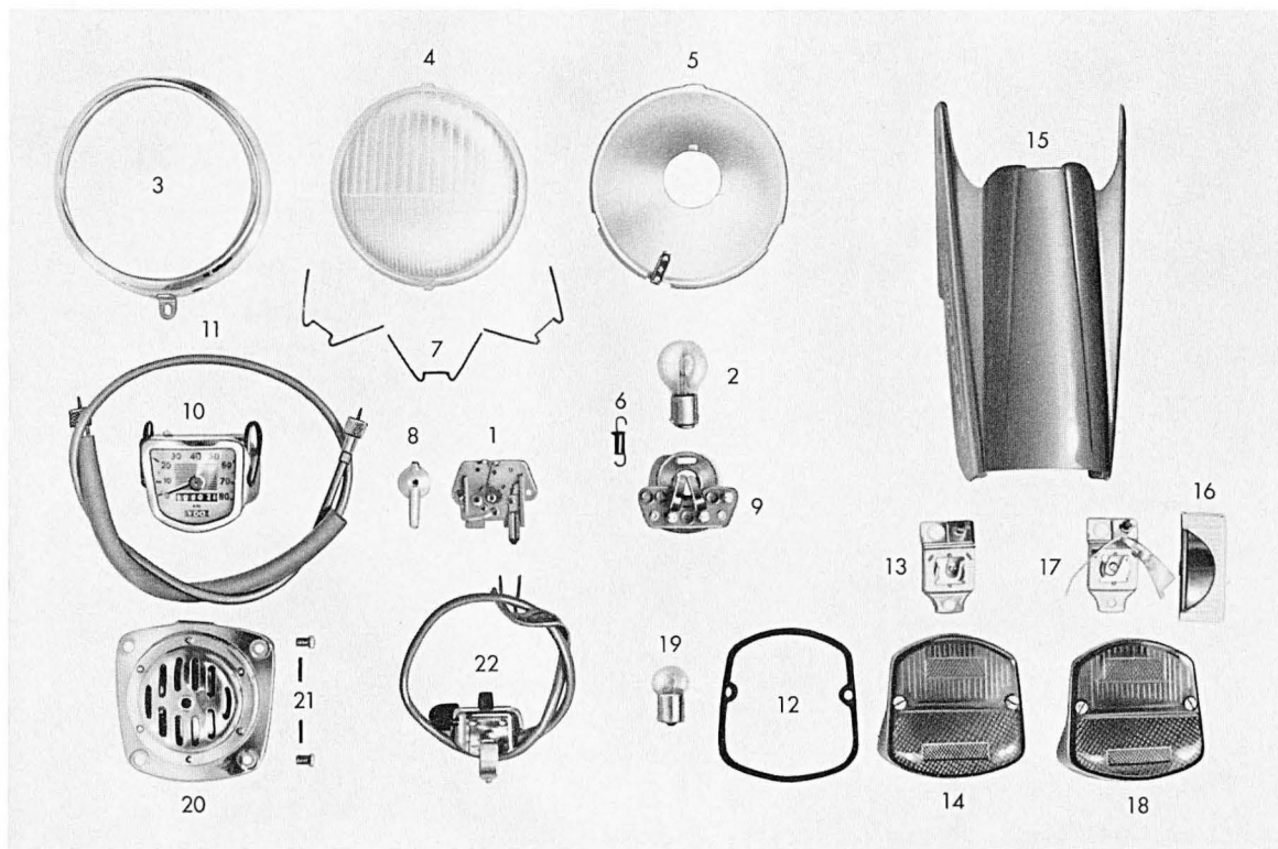
Tafel 7/1 Lichtanlage - Tachometer - Rücklicht (Bilux)
