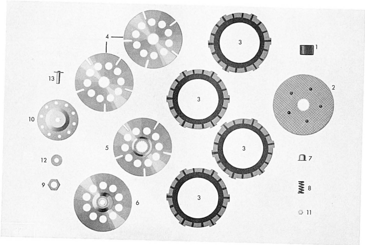
Tafel 10 a Kupplung
