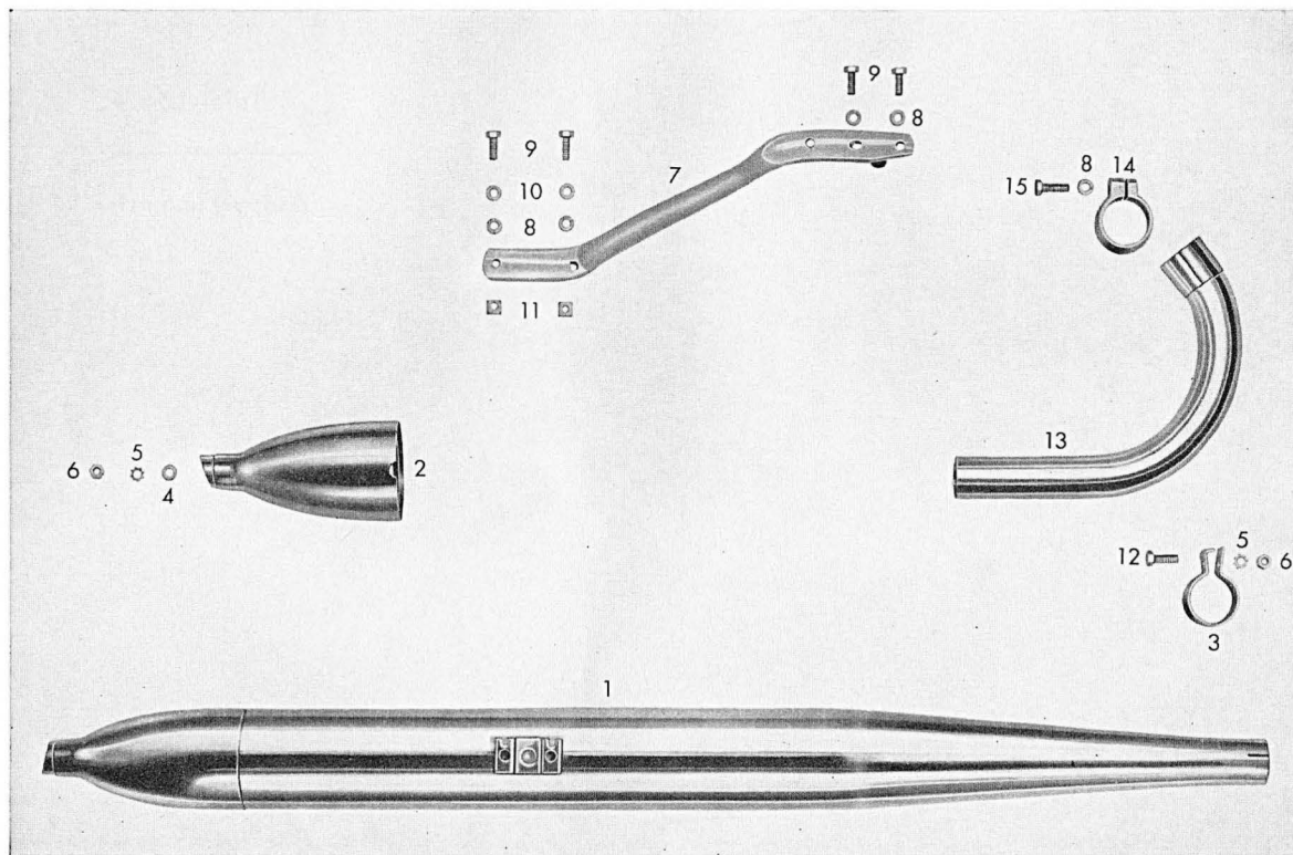
Tafel 12 a/1 Auspuff (Export)
