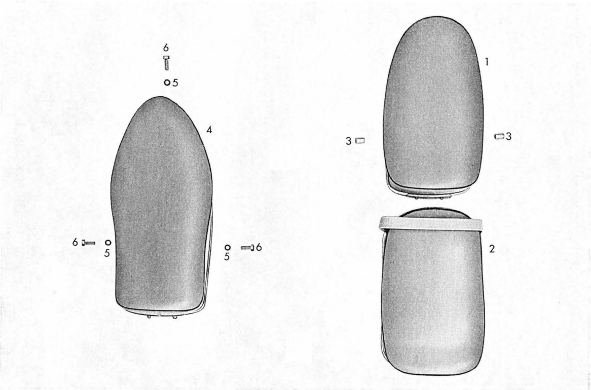
Tafel 13 Sitzkissen - Einzelsitzbank
