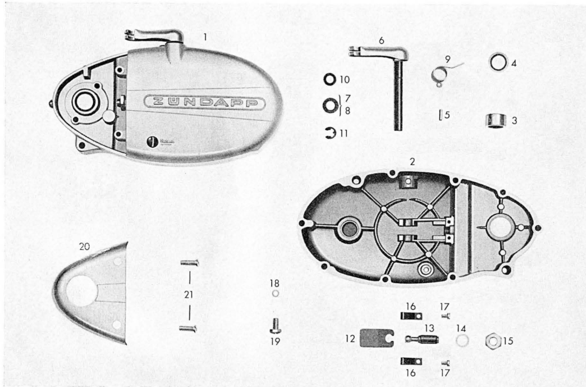
Tafel 4 Gehäusedeckel rechts
