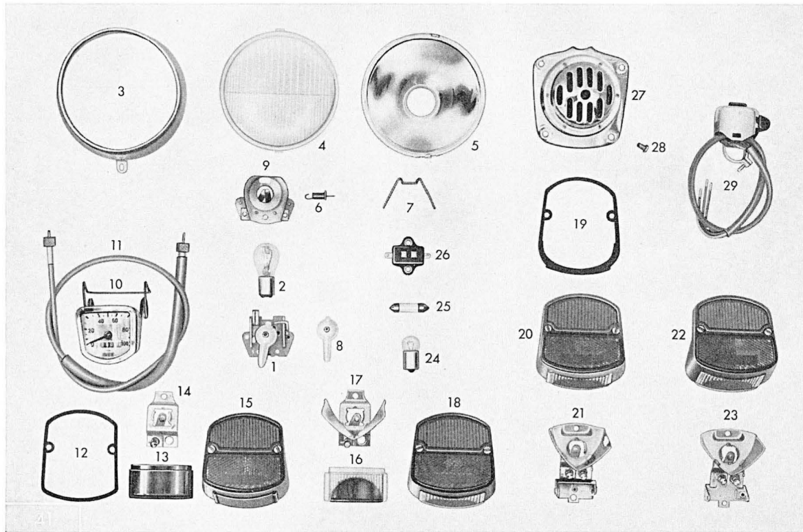
Tafel 7a/1 Lichtenanlage – Tachometer – Rücklicht (Bilux)
