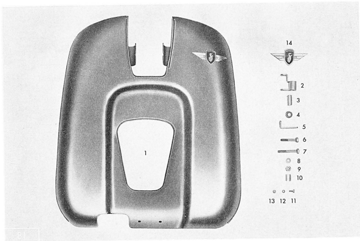
Tafel 14 a Beinschild
