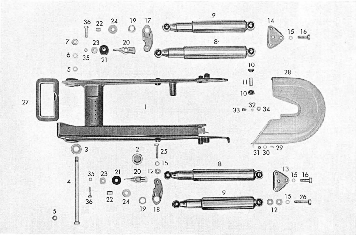
Tafel 4 Hinterradgabel - Federbein
