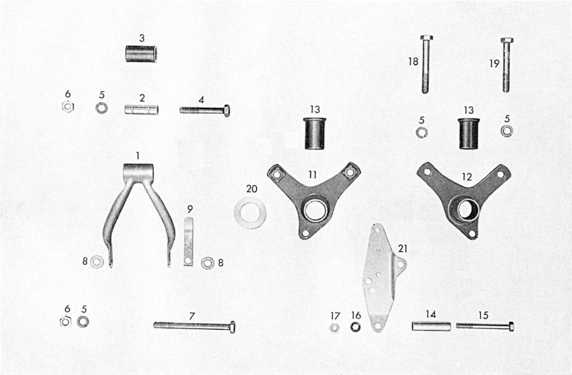
Tafel 2 Motoraufhängung
