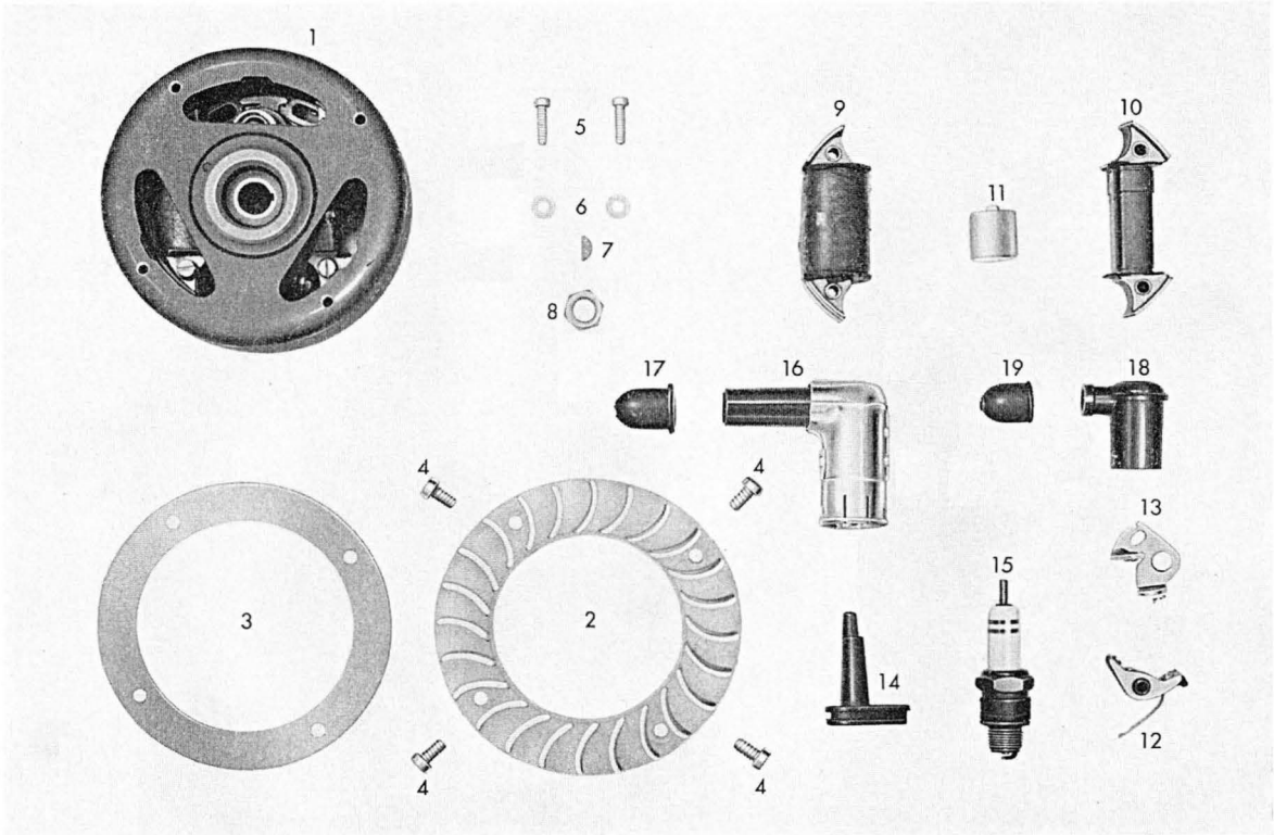
Tafel 11/1 Elektrische Ausrüstung (nur für Motor mit Gebläse)
