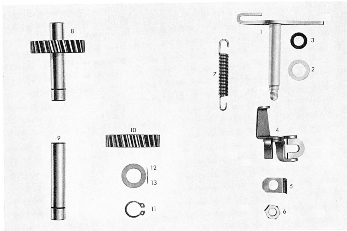
Tafel 8 Schalthebel-Schaltgabel-Welle z. Zwischenrad
