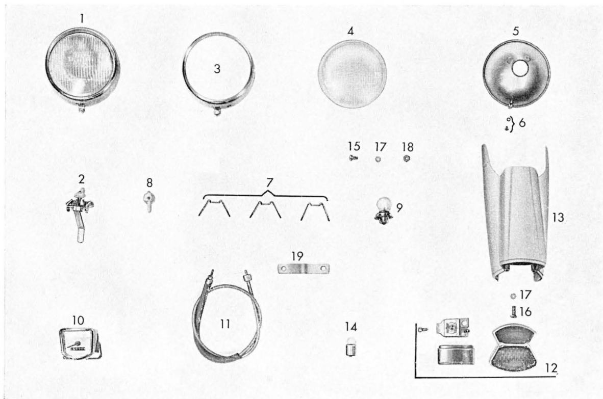
Tafel 7 Lichtanlage - Tachometer - Rücklicht
