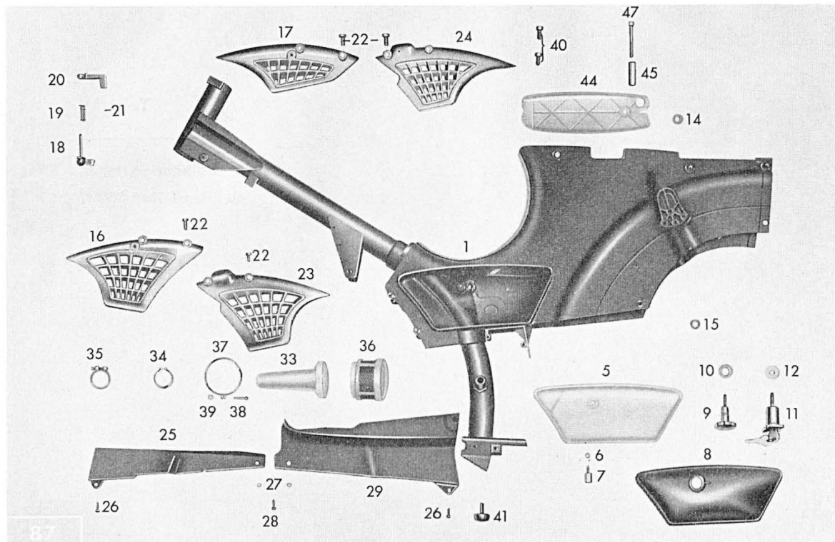
Tafel 1 c Rahmen – Mittelteil
