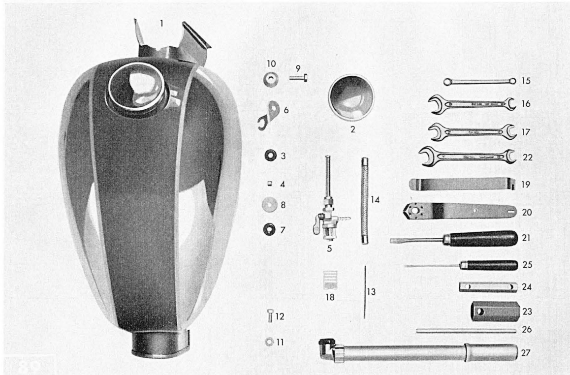
Tafel 10 a Kraftstoffbehälter – Werkzeuge
