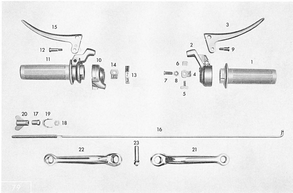
Tafel 8 c Schalt-, Betätigungshebel – Züge (Handschtaltung)
