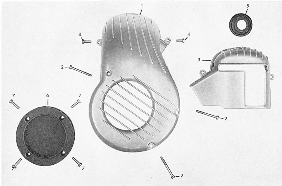
Tafel 3 b Lüftergehäuse – Lüfterrad
