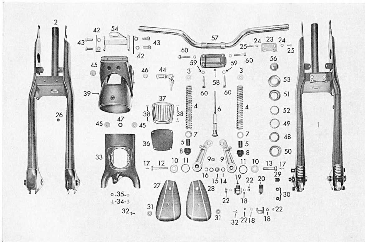
Tafel 3 a Vorderradgabel - Lenkungslager - Scheinwerfergehäuse
