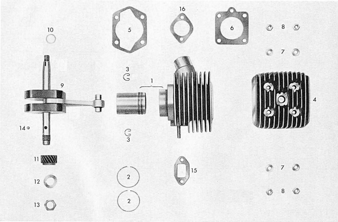
Tafel 5/1 Zylinder-Kurbeltrieb (nur für Motore mit Gebläse)
