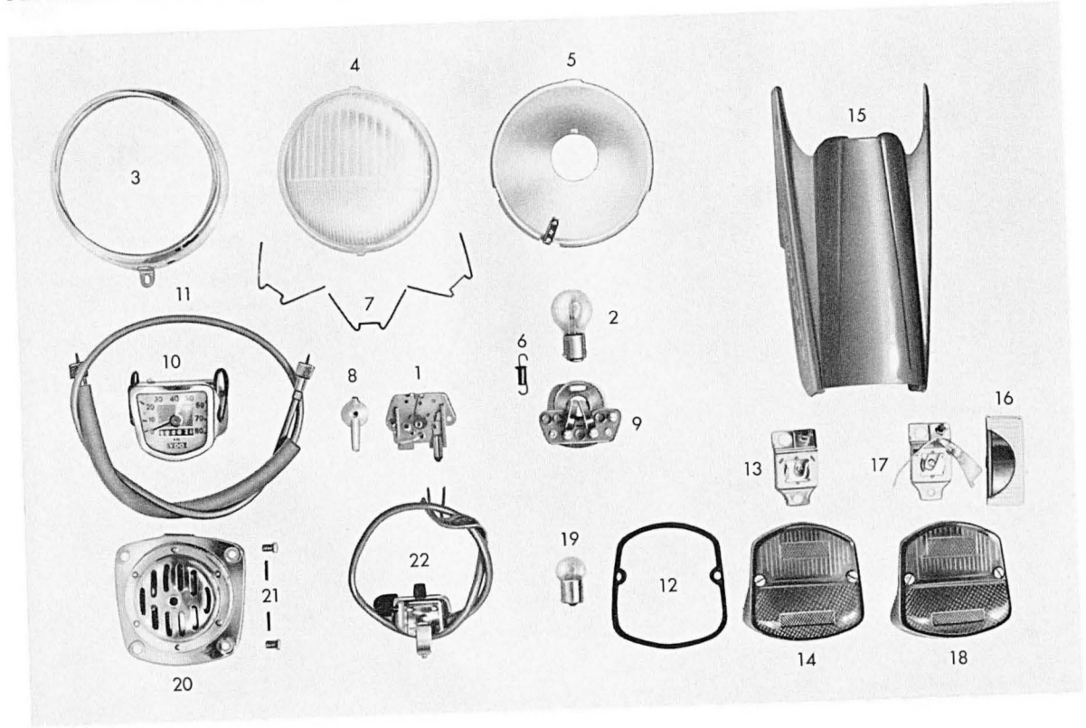
Tafel 7/1 Lichtanlage - Tachometer - Rücklicht (Bilux)
