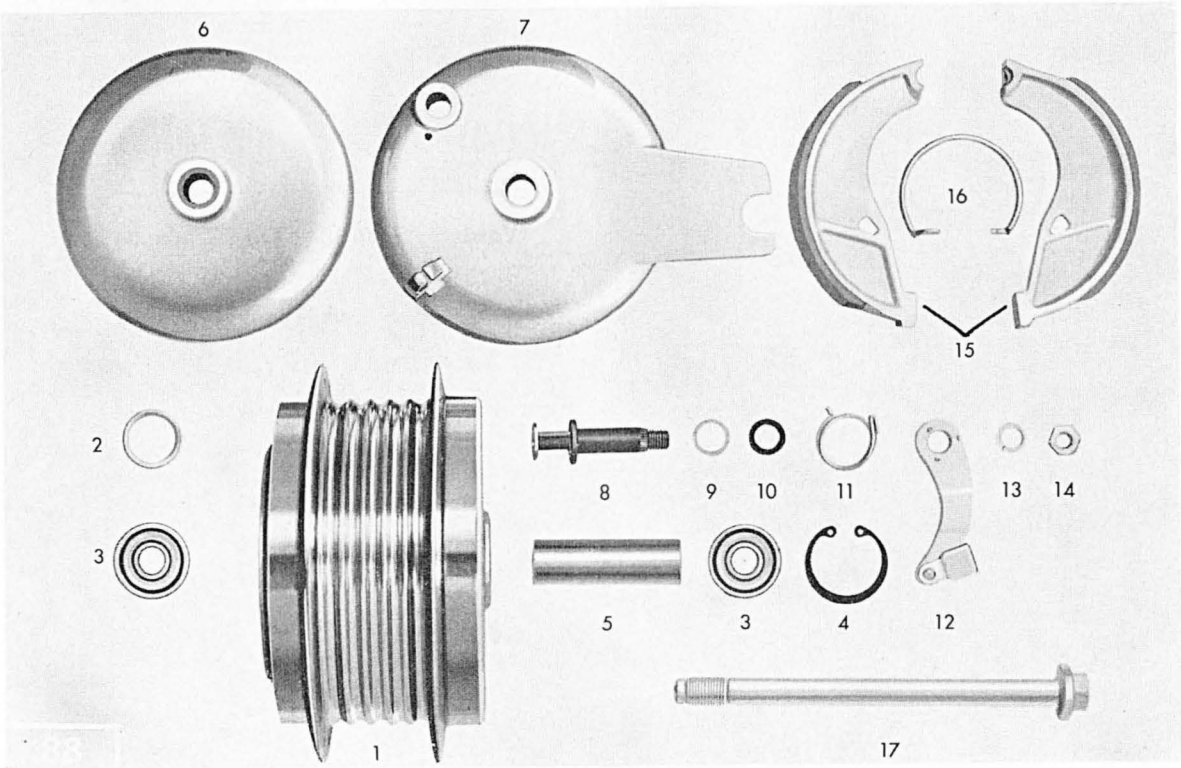
Tafel 5 b Vorderes Laufrad – Vorderradnabe 21"-Räder
