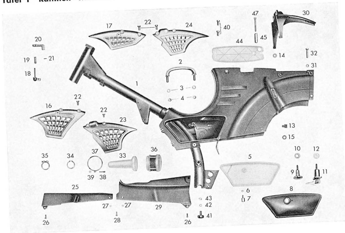
Tafel 1 Rahmen - Mittelteil
