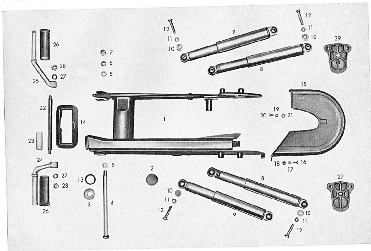
Tafel 4 b Hinterradgabel – Federbein, Fußrasten
