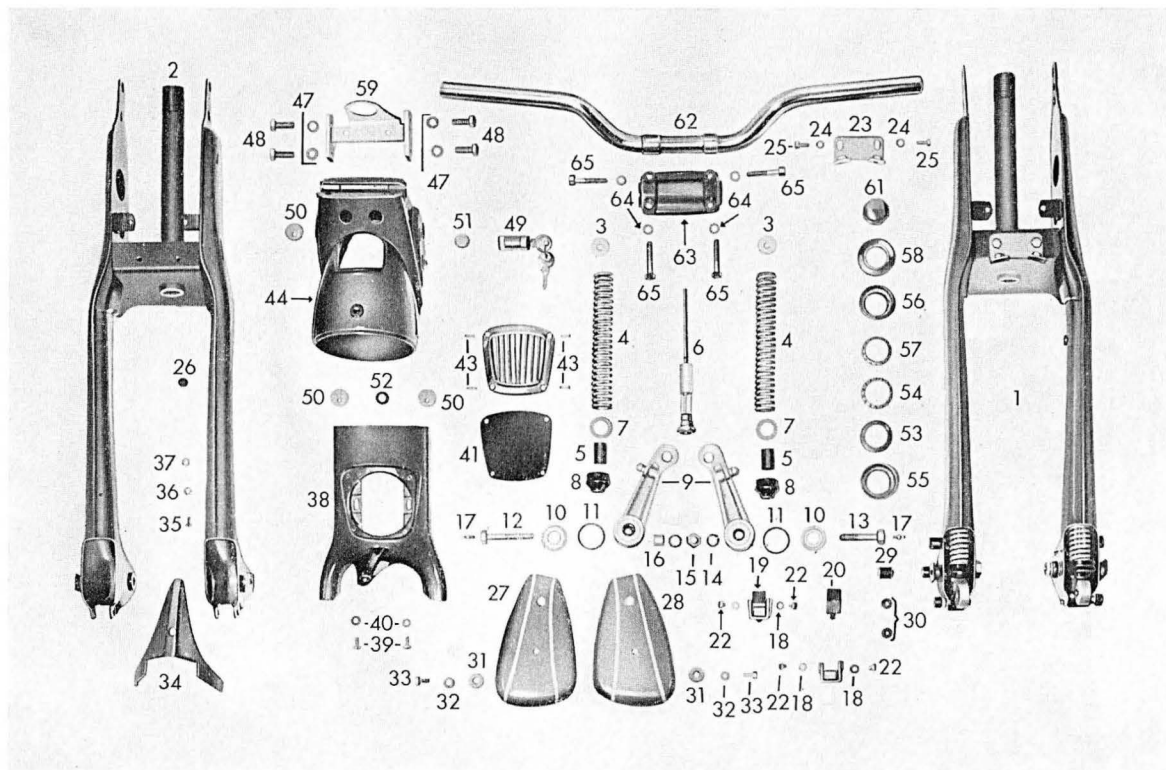
Tafel 3 Vorderradgabel - Lenkungslager - Scheinwerfergehäuse
