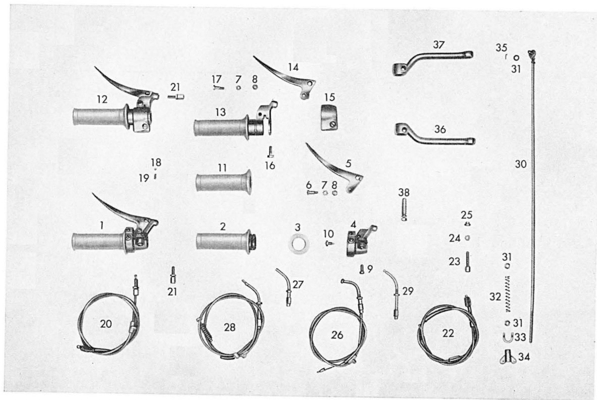
Tafel 8 b Schalt-, Betätigungshebel – Züge
