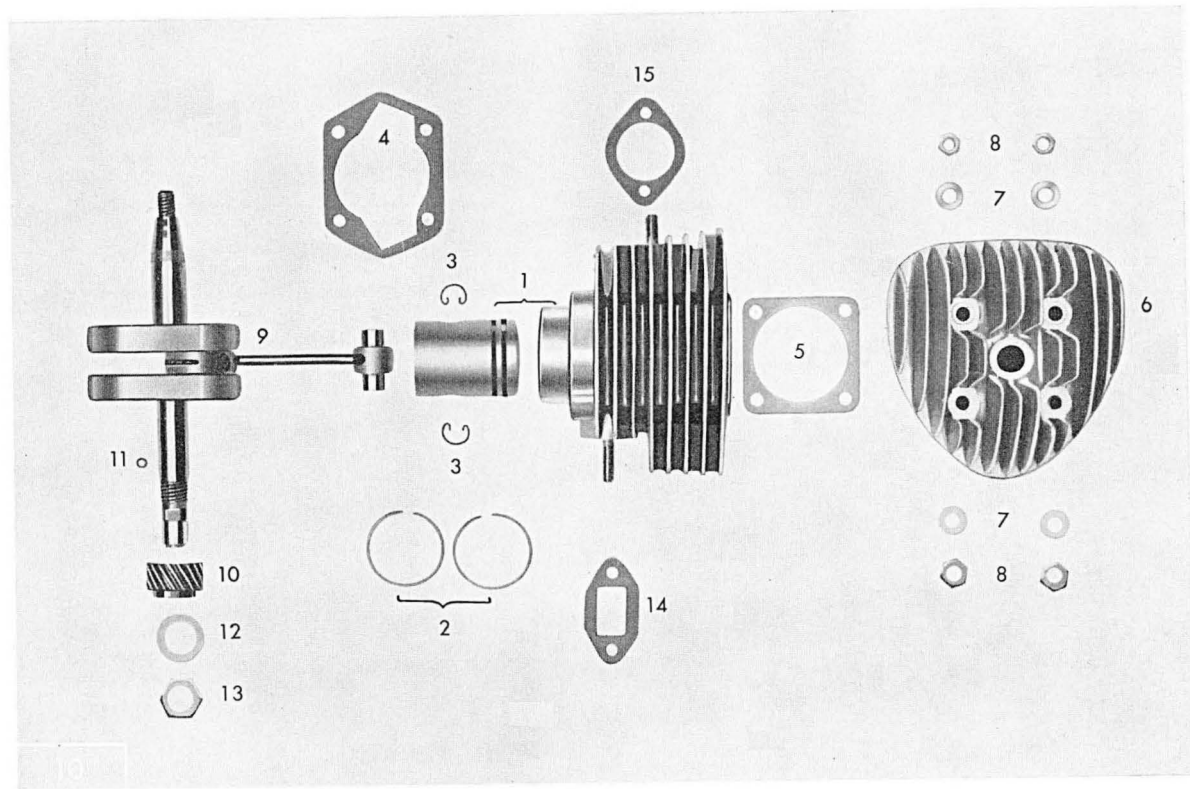
Tafel 5 c Zylinder – Kurbeltrieb (nur für Motoren ohne Gebläse)
