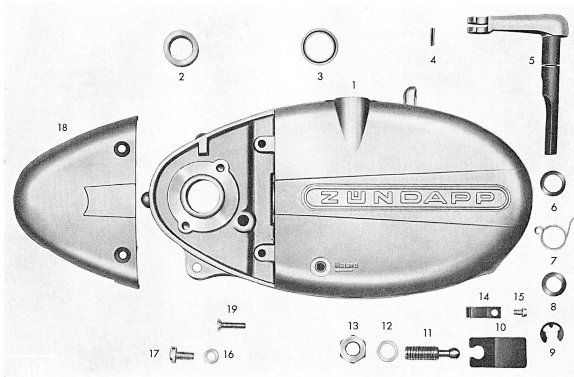
Tafel 4 b Gehäusedeckel rechts
