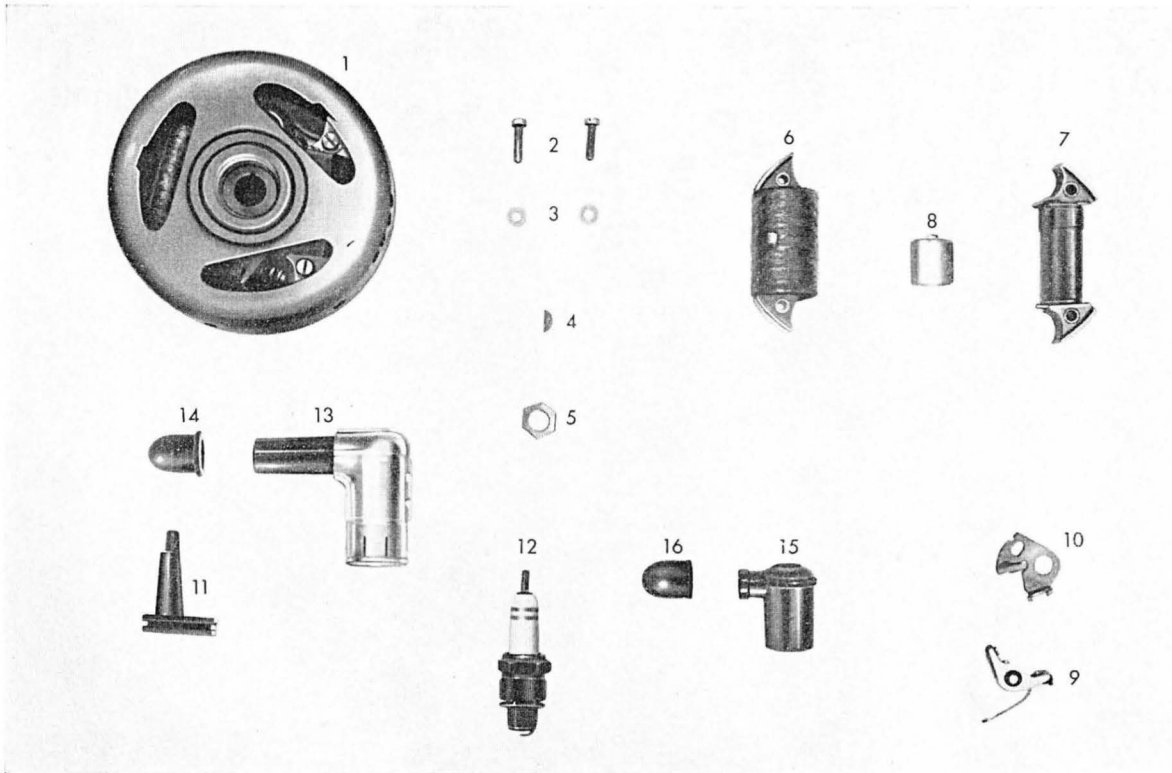
Tafel 11 Elektrische Ausrüstung (nur für Motor ohne Gebläse)
