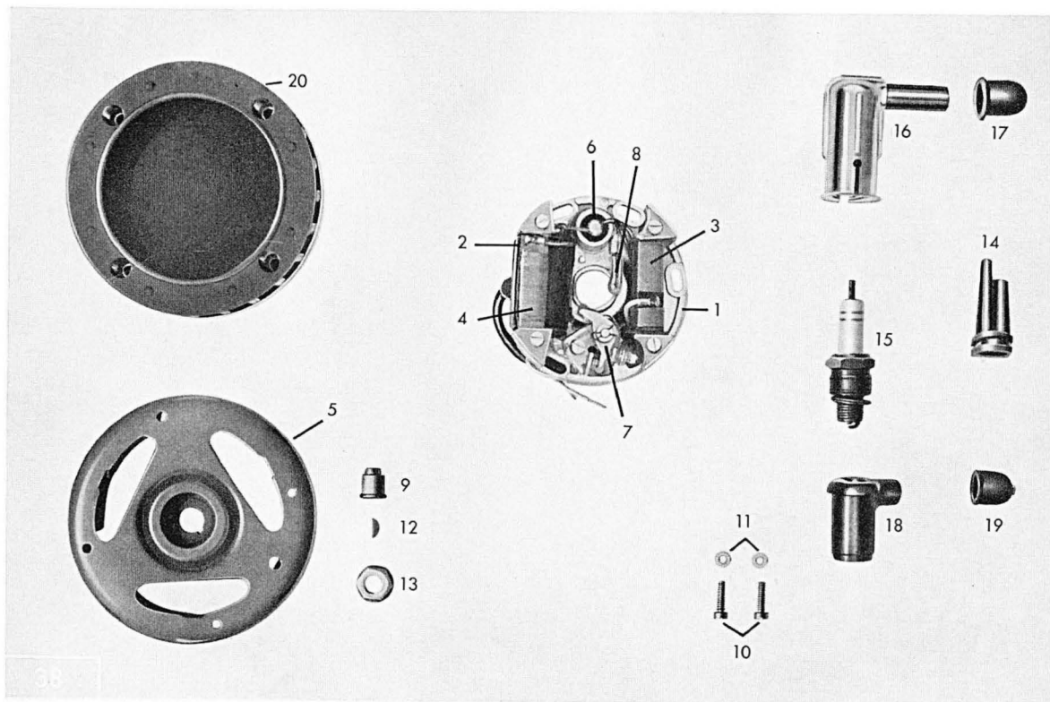
Tafel 11 a/1 Elektrische Ausrüstung
