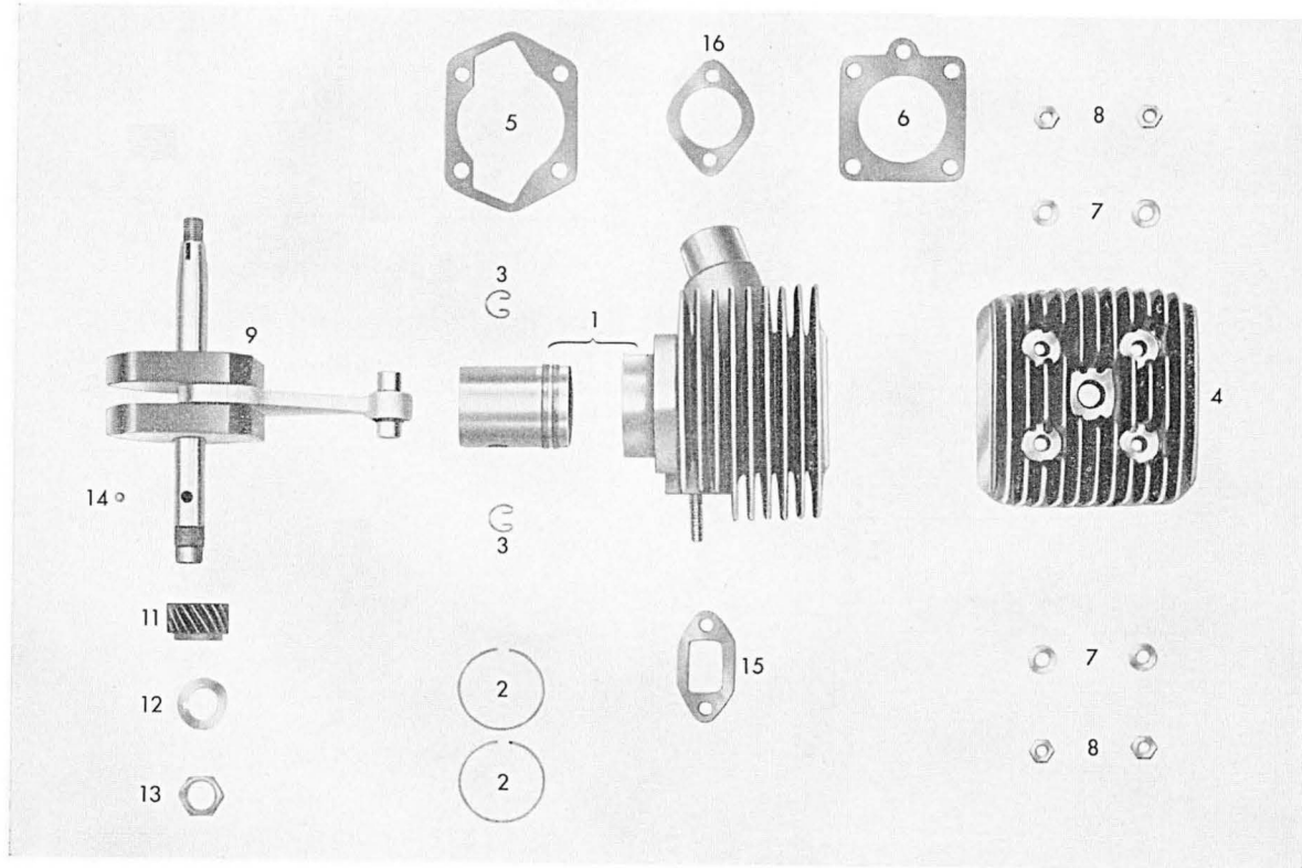
Tafel 5 a/1 Zylinder - Kurbeltrieb (nur für Motoren mit Gebläse)
