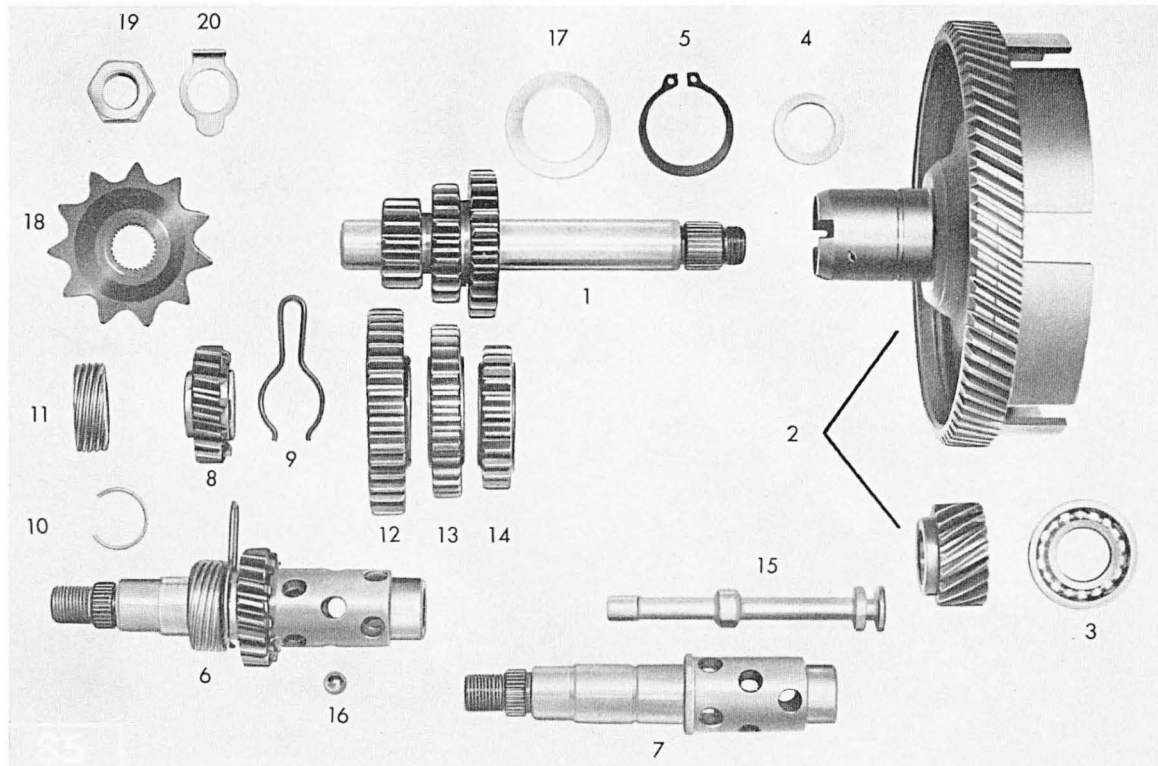
Tafel 7 b Getriebe – Schaltwelle
