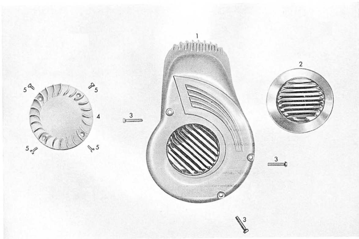
Tafel 3 Lüftergehäuse - Lüfterrad
