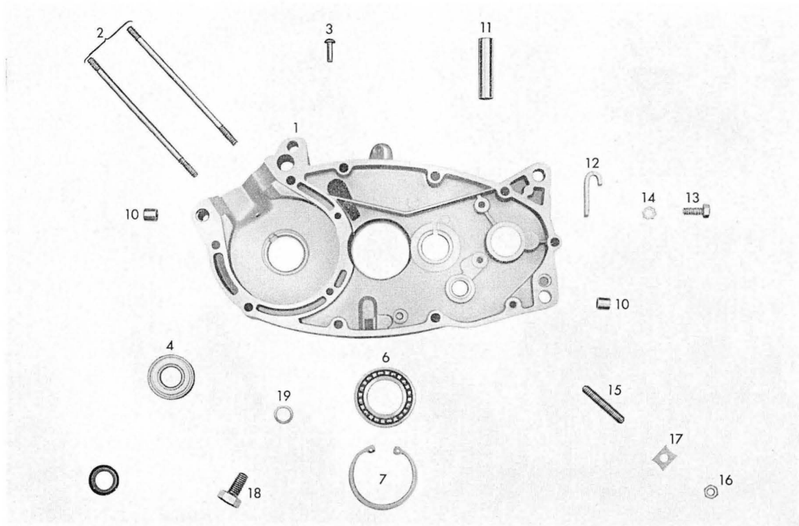
Tafel 1 a Gehäusehälfte rechts
