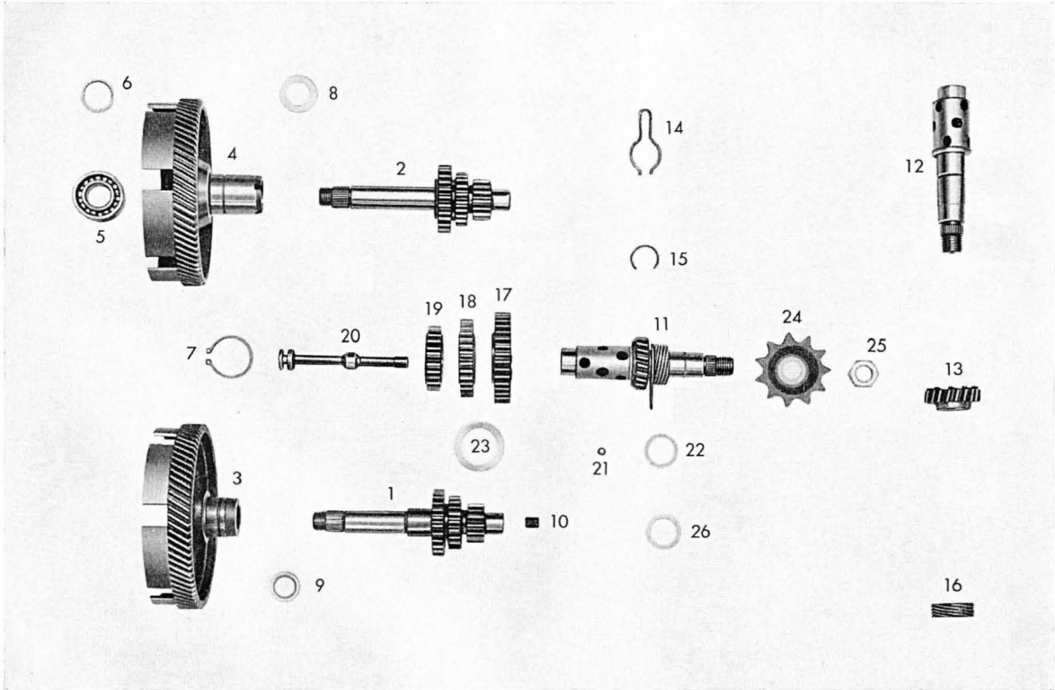
Tafel 7 Getriebe-Schaltwelle
