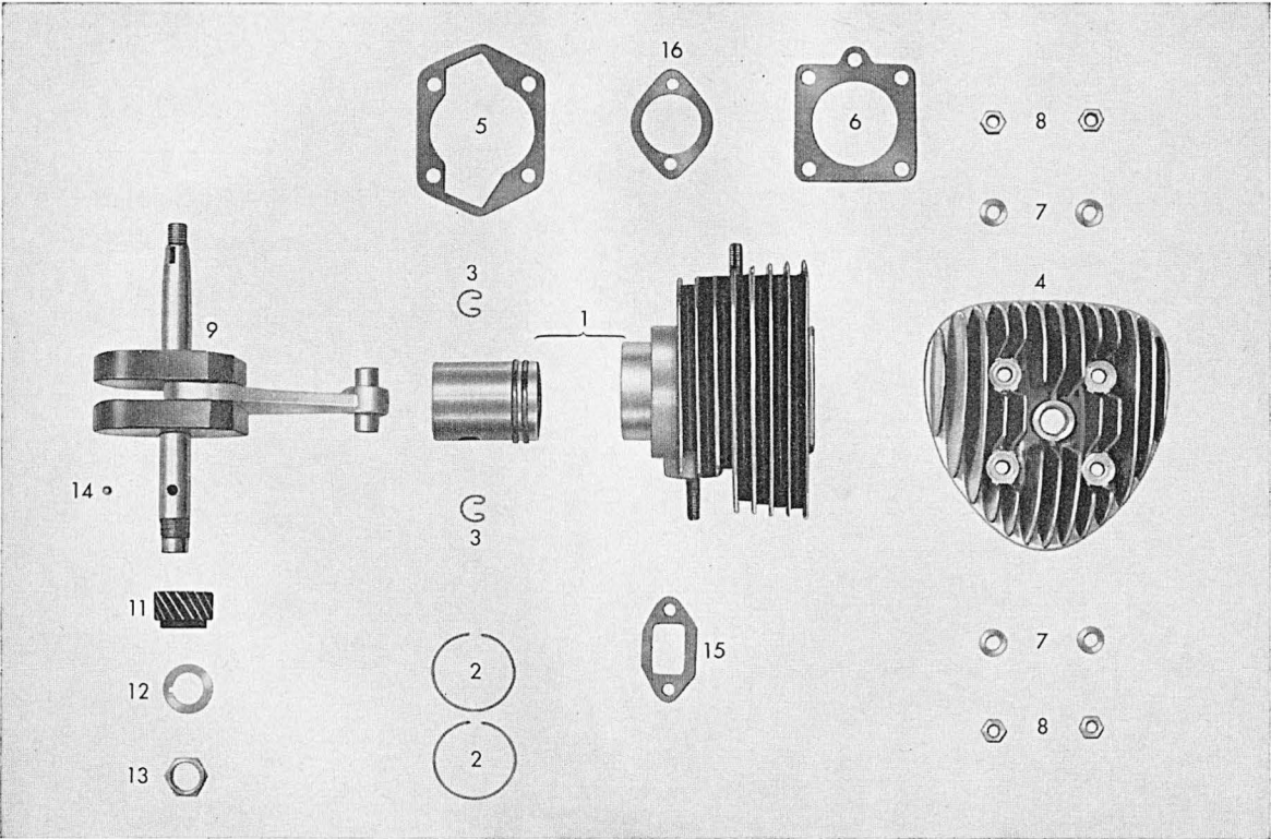
Tafel 5 b Zylinder-Kurbeltrieb (nur für Motoren ohne Gebläse)
