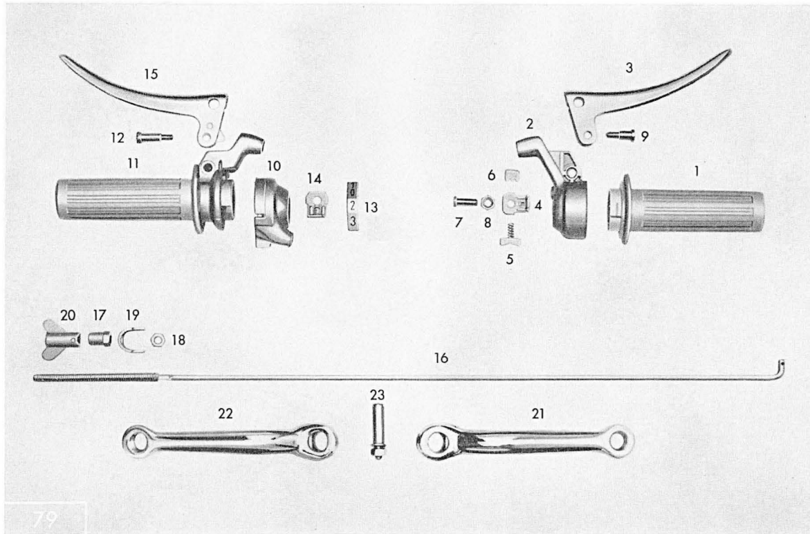
Tafel 8 c Schalt-, Betätigungshebel – Züge (Handschaltung)
