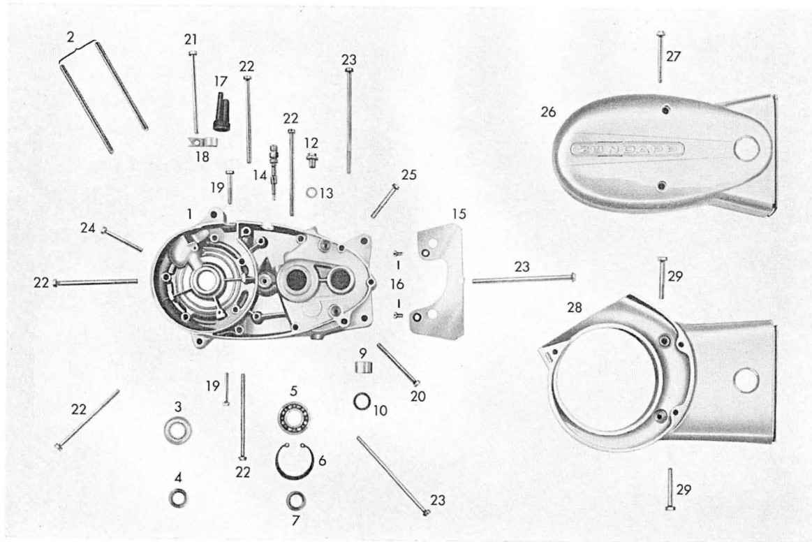
Tafel 2 c Gehäusehälfte links
