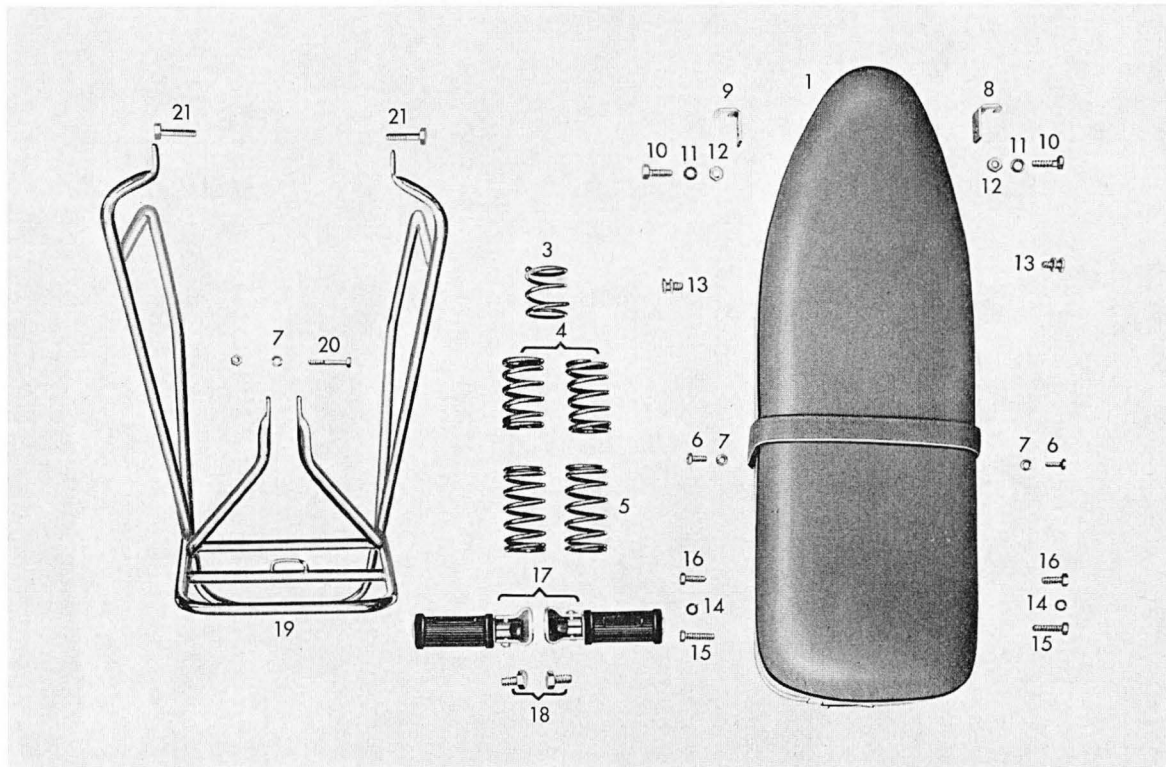
Tafel 12 Doppelsitzbank
