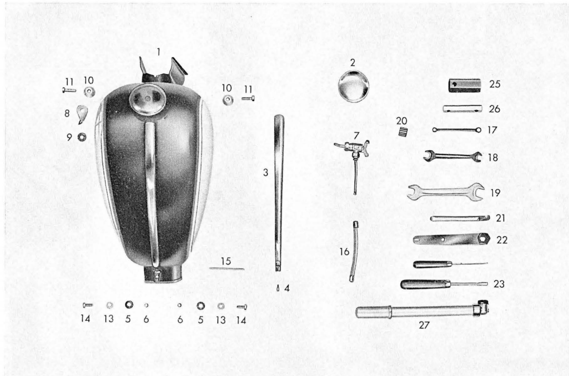
Tafel 10 Kraftstoffbehälter - Werkzeuge
