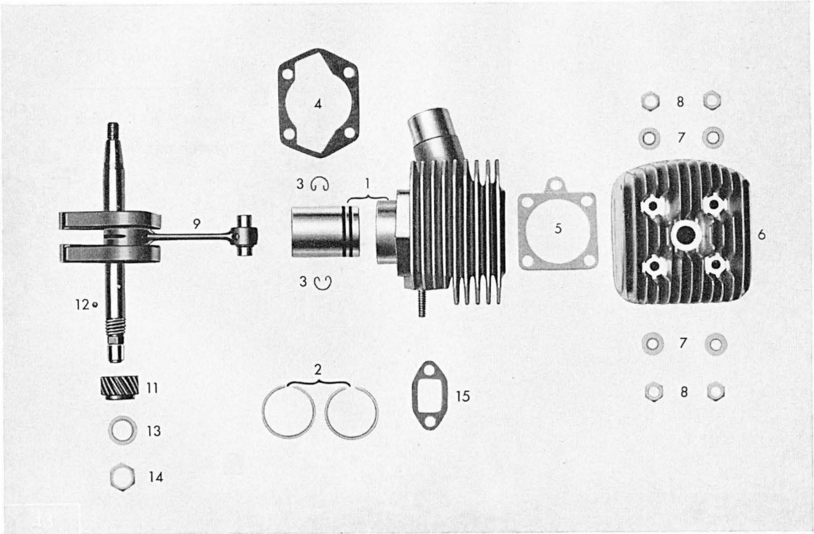
Tafel 5 b/1 Zylinder-Kurbeltrieb (nur für Motoren mit Gebläse)
