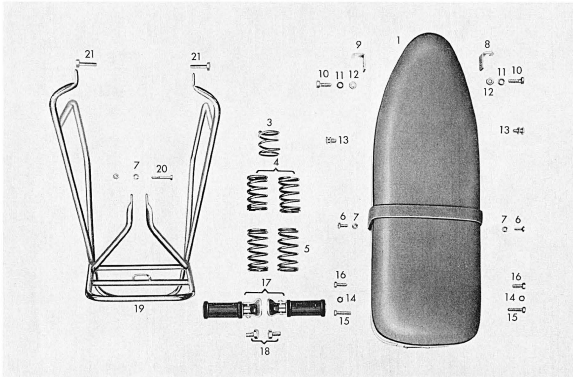
Tafel 12 Doppelsitzbank
