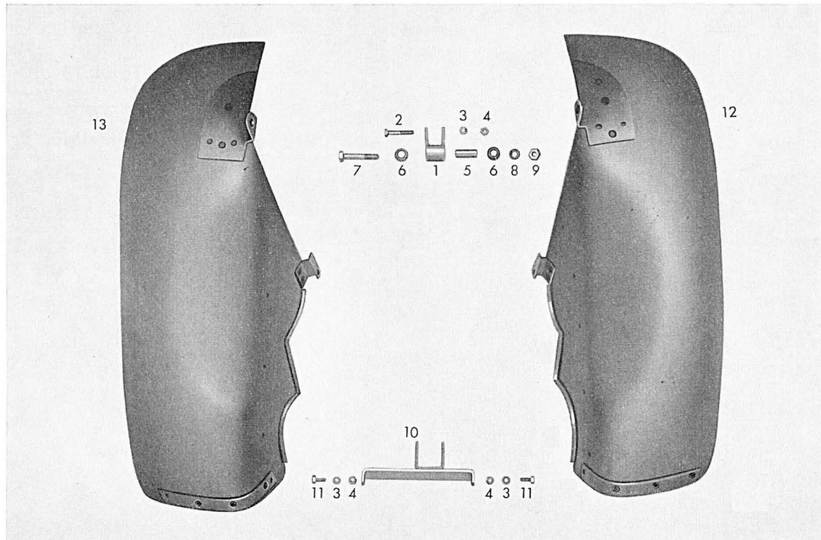
Tafel 14 Beinschild
