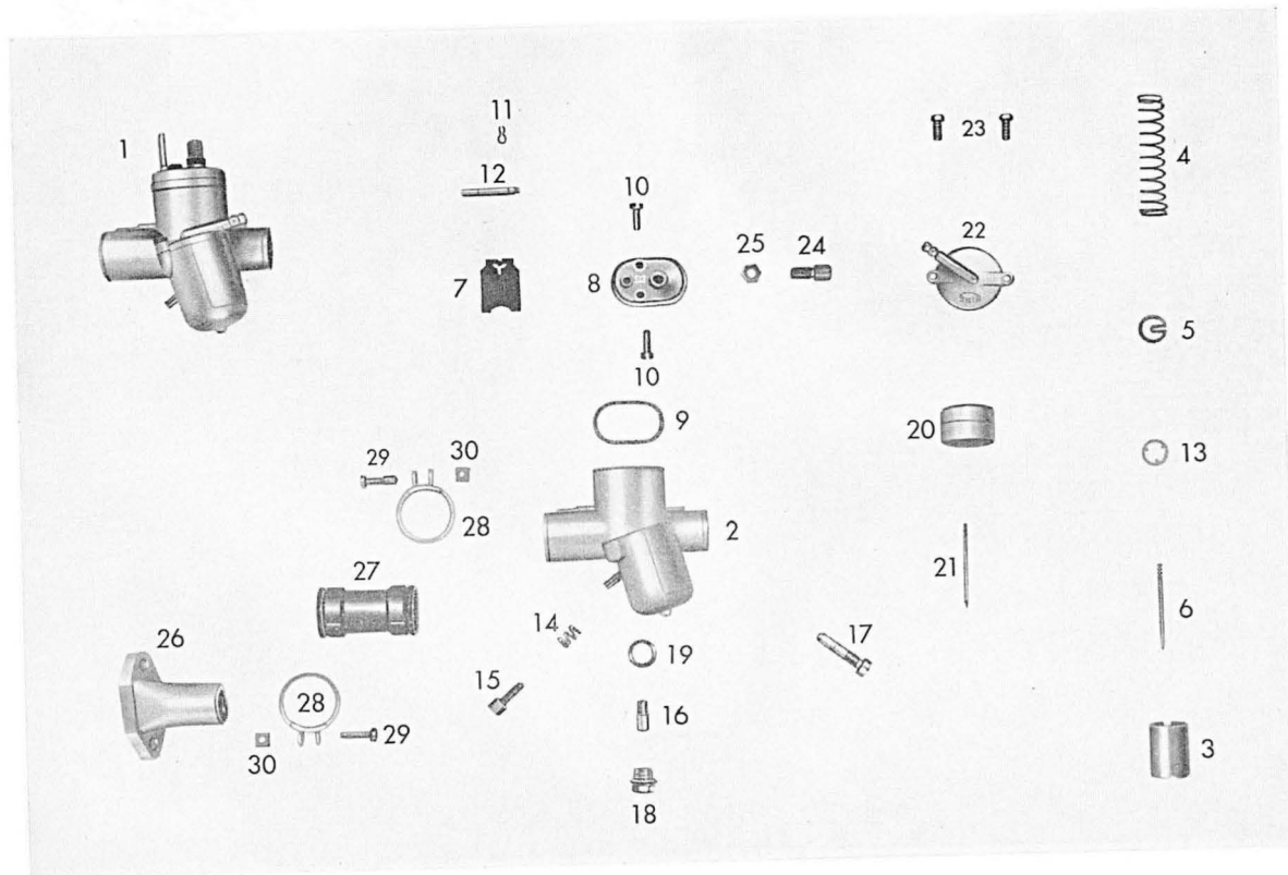
Tafel 6 a Vergaser
