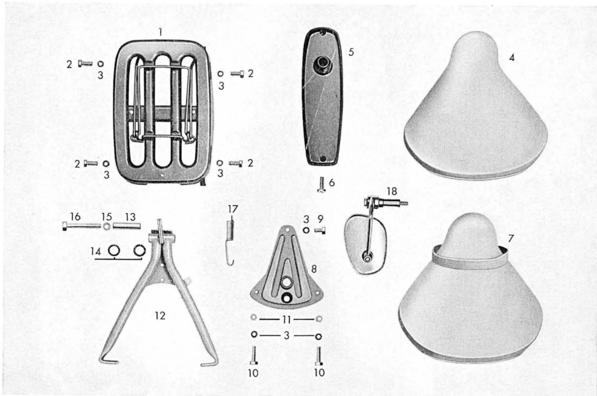
Tafel 11 Gepäckträger - Sattel - Radständer
