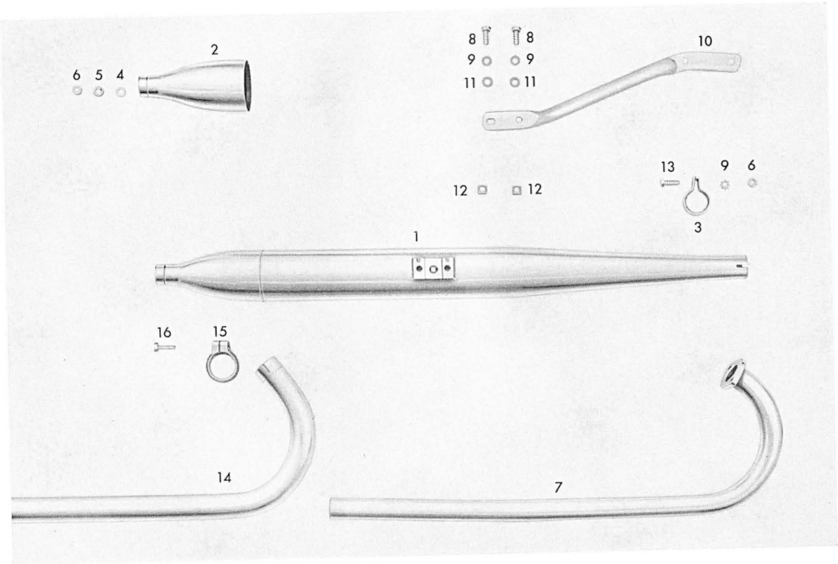
Tafel 12 a Auspuff
