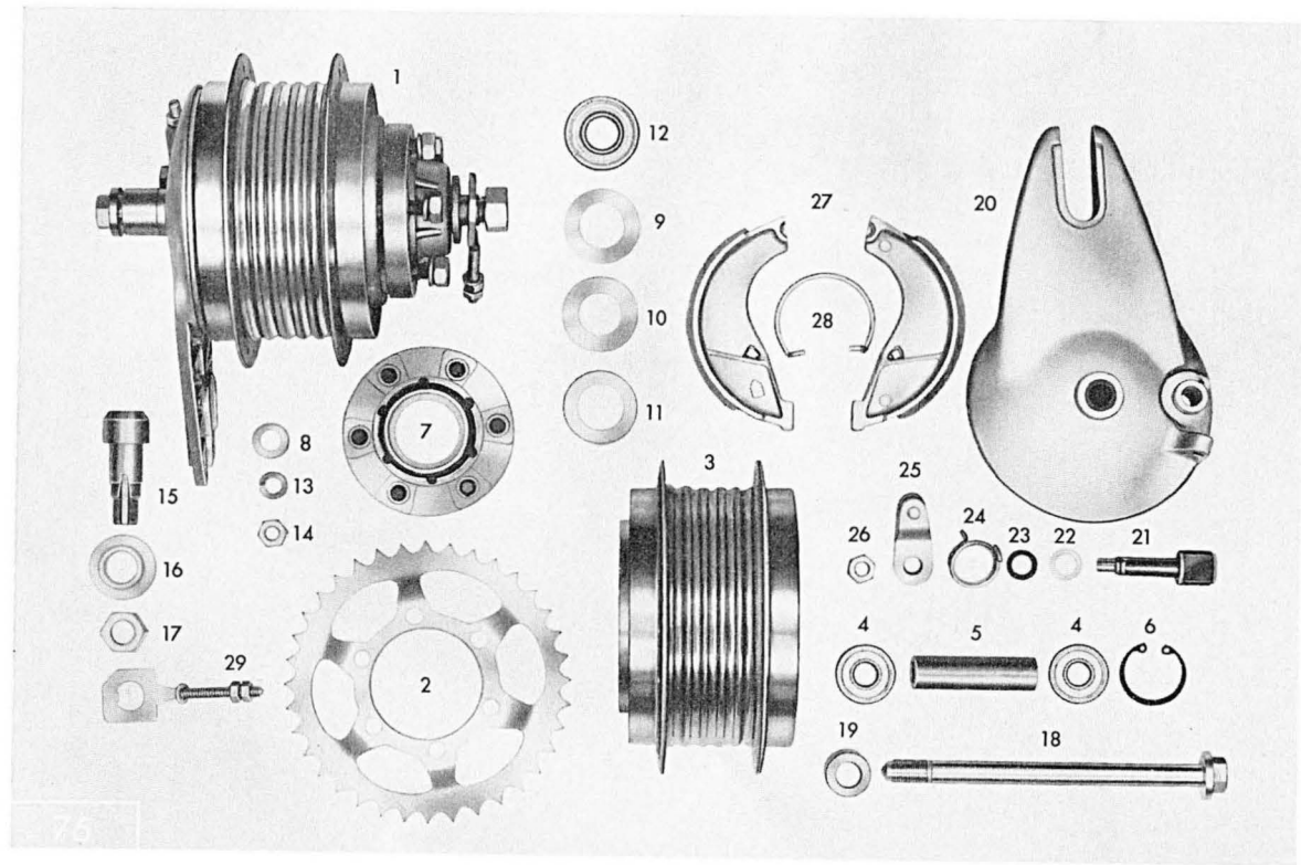
Tafel 6 b Hinteres Laufrad – Hinterradnabe 21"-Räder
