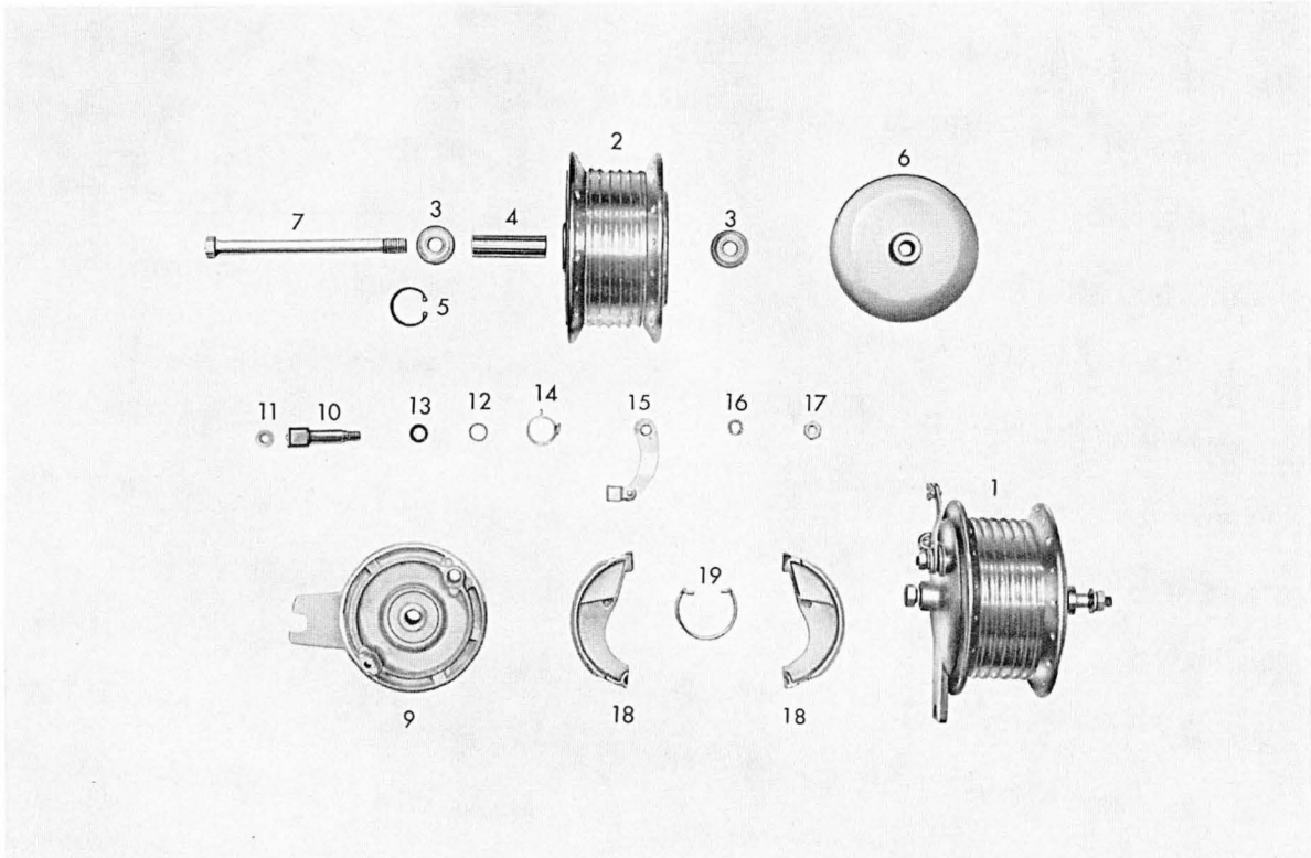
Tafel 5 a Vorderes Laufrad - Vorderradnabe
