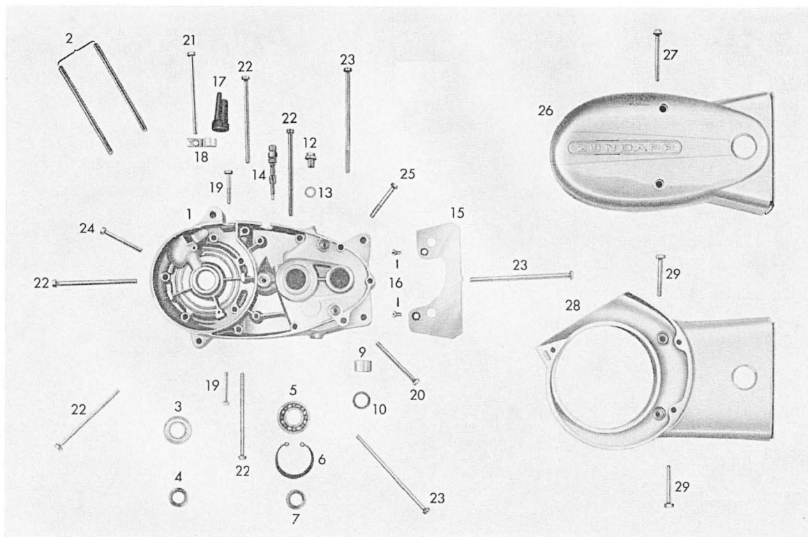
Tafel 2 a Gehäusehälfte links
