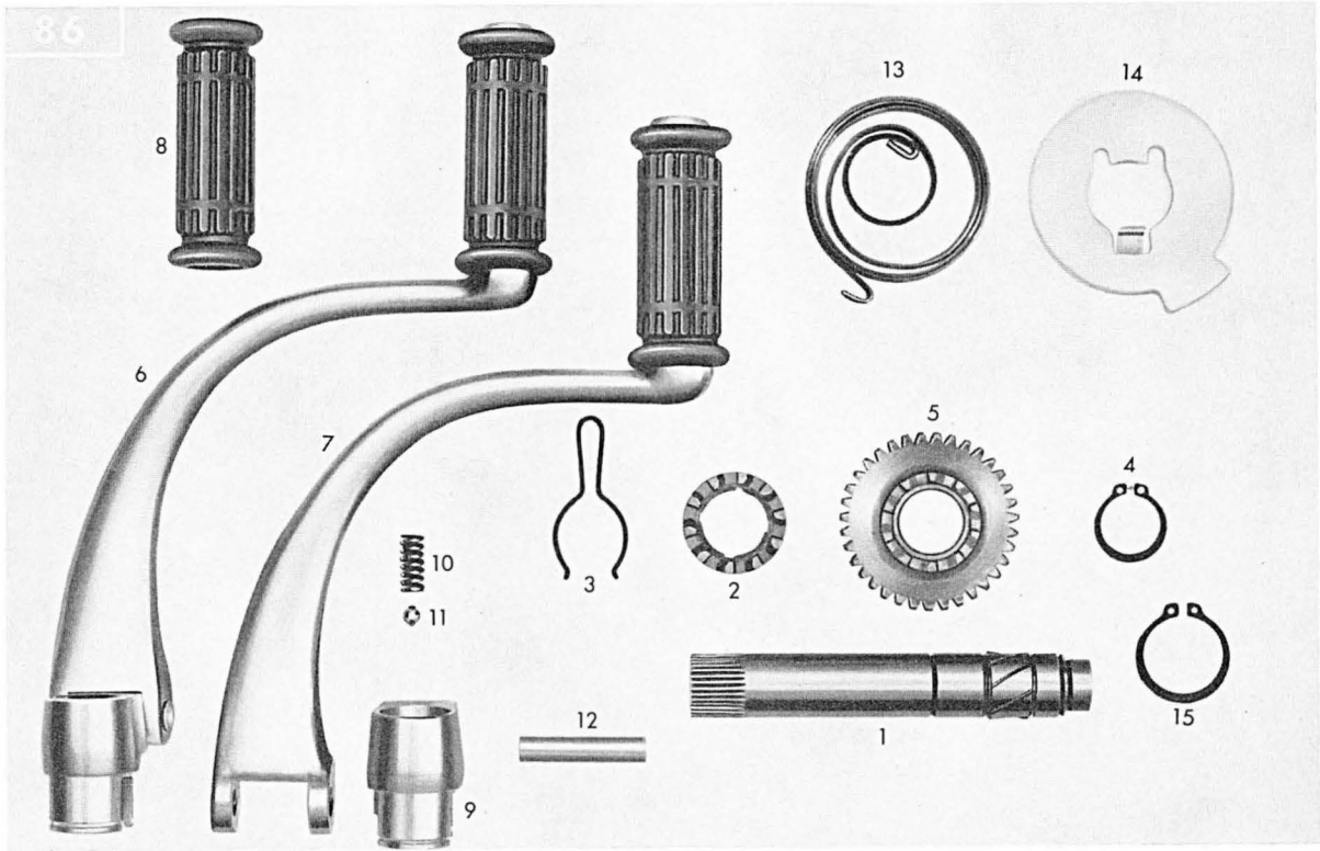
Tafel 9/1 a Kickstarterwelle – Kickstarterhebel
