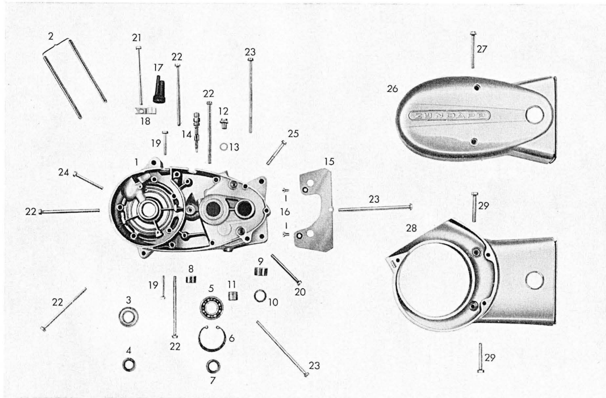
Tafel 2 Gehäusehälfte links
