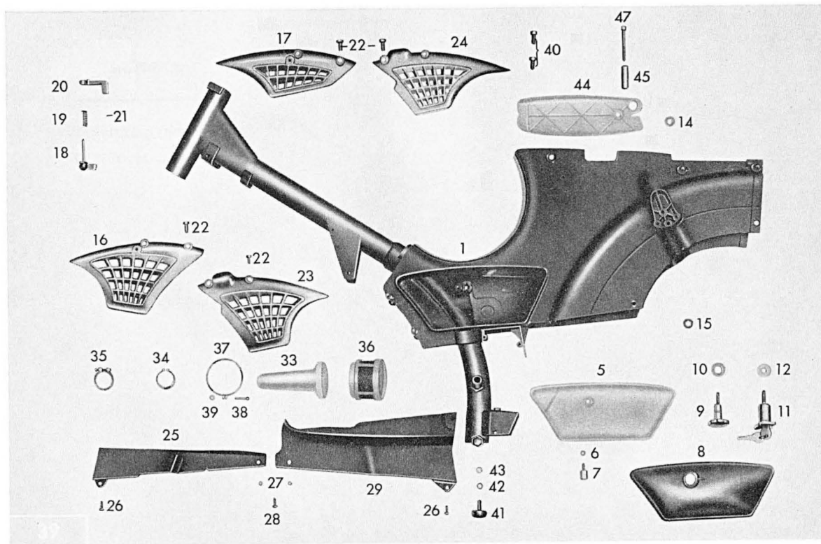
Tafel 1 b Rahmen – Mittelteil
