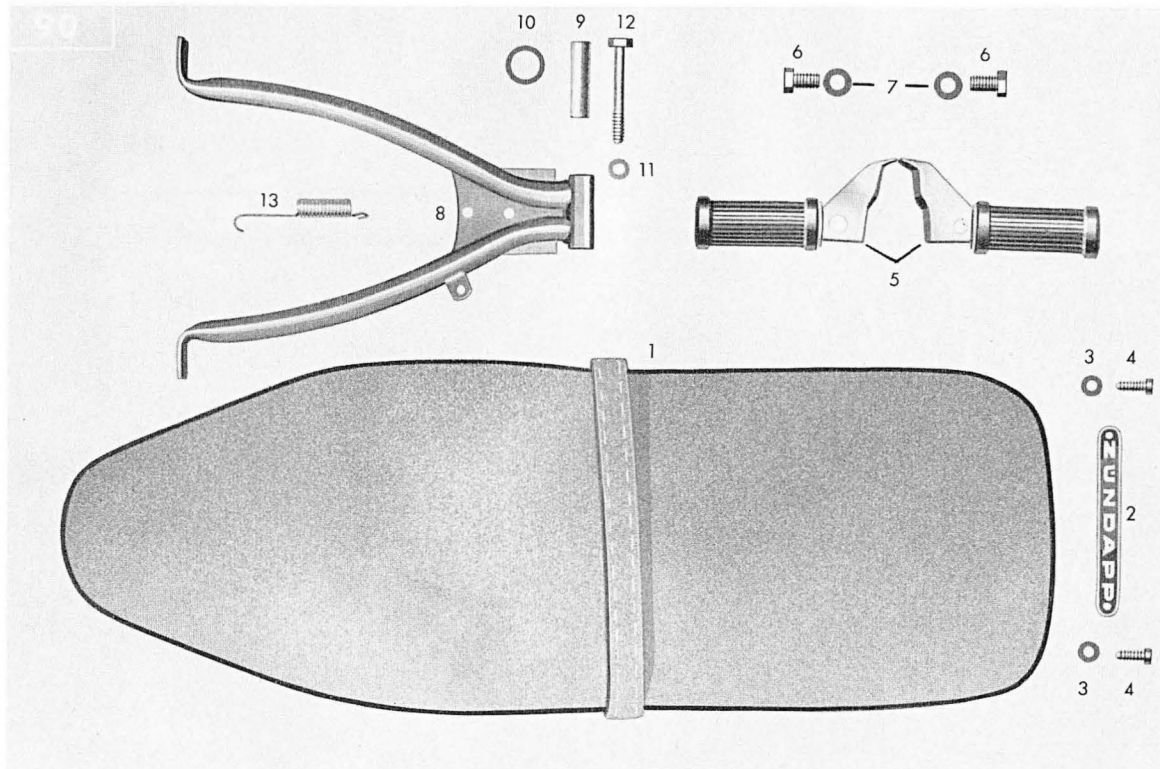
Tafel 12 b Doppelsitzbank – Radständer
