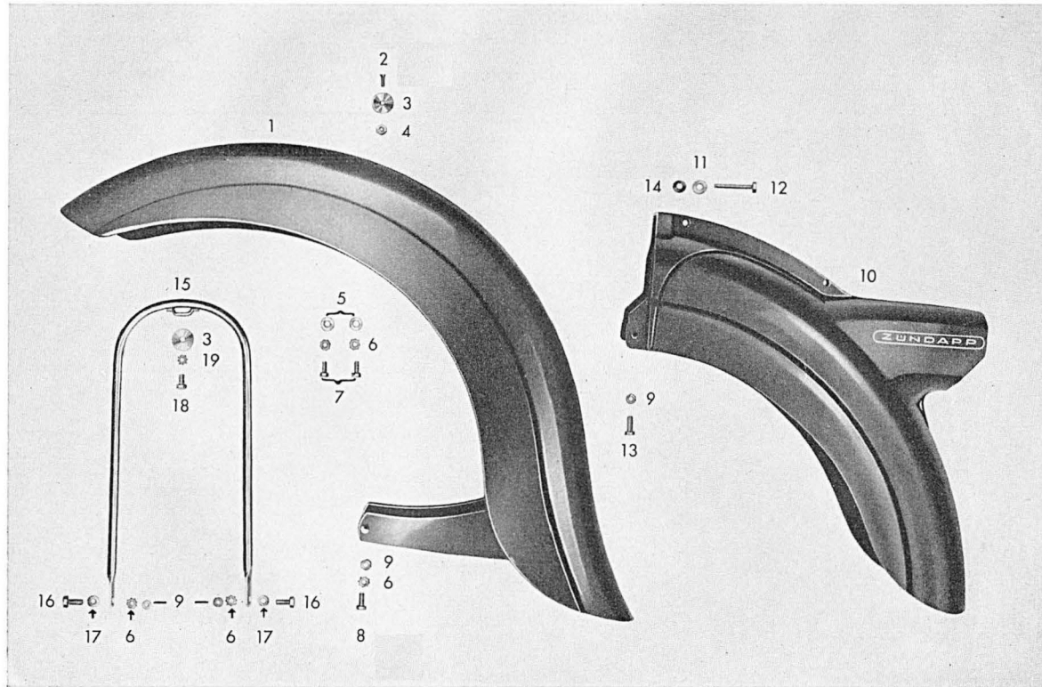
Tafel 9 b Schutzblech – Rahmen-Endteil – Zierbügel
