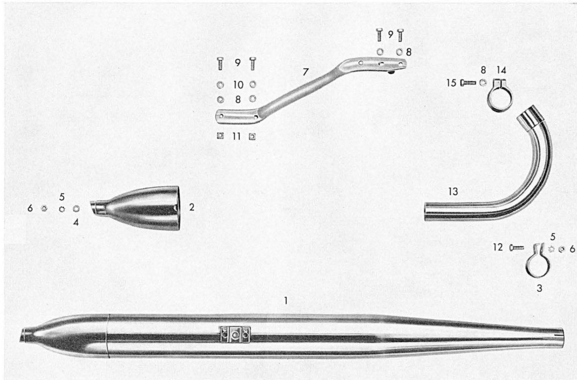
Tafel 12 b/1 Auspuff (Export)
