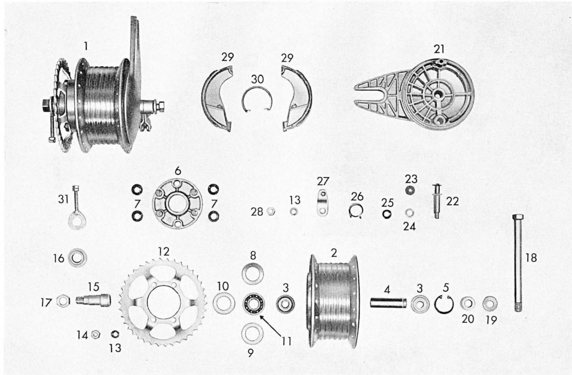
Tafel 6 a Hinteres Laufrad - Hinterradnabe
