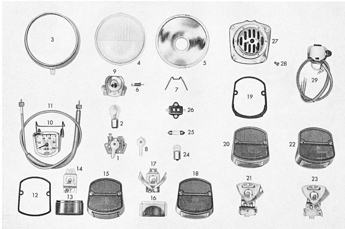
Tafel 7a/1 Lichtanlage – Tachometer – Rücklicht (Bilux)
