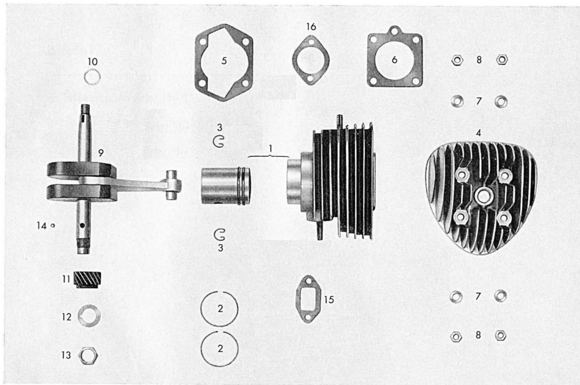
Tafel 5 Zylinder-Kurbeltrieb (nur für Motore ohne Gebläse)
