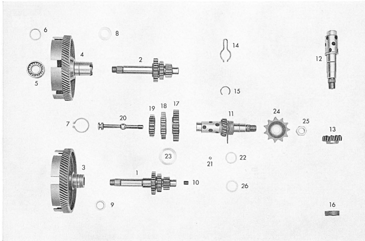
Tafel 7 a Getriebe-Schaltwelle
