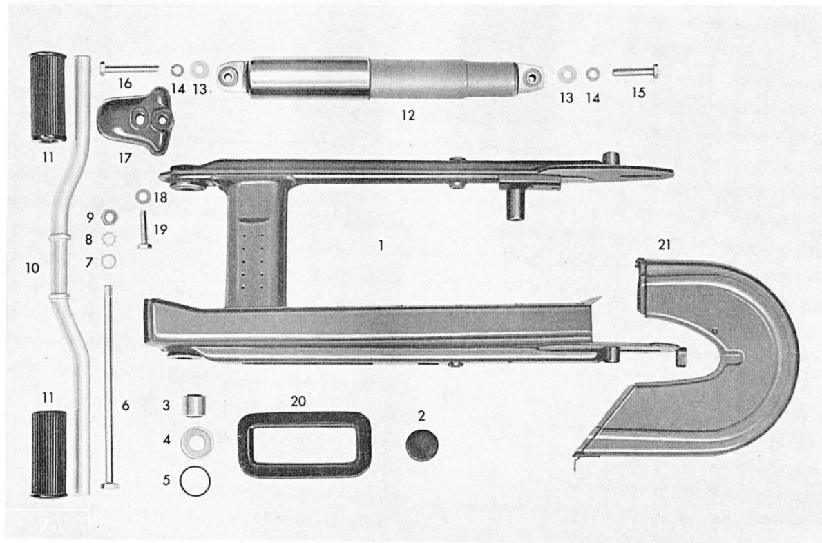
Tafel 4 c Hinterradgabel – Federbein – Fußrastenrohr
