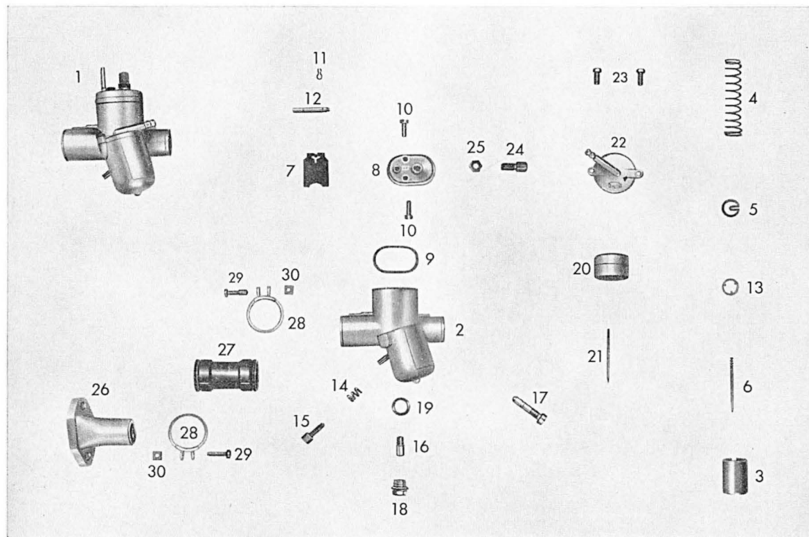
Tafel 6 b Vergaser
