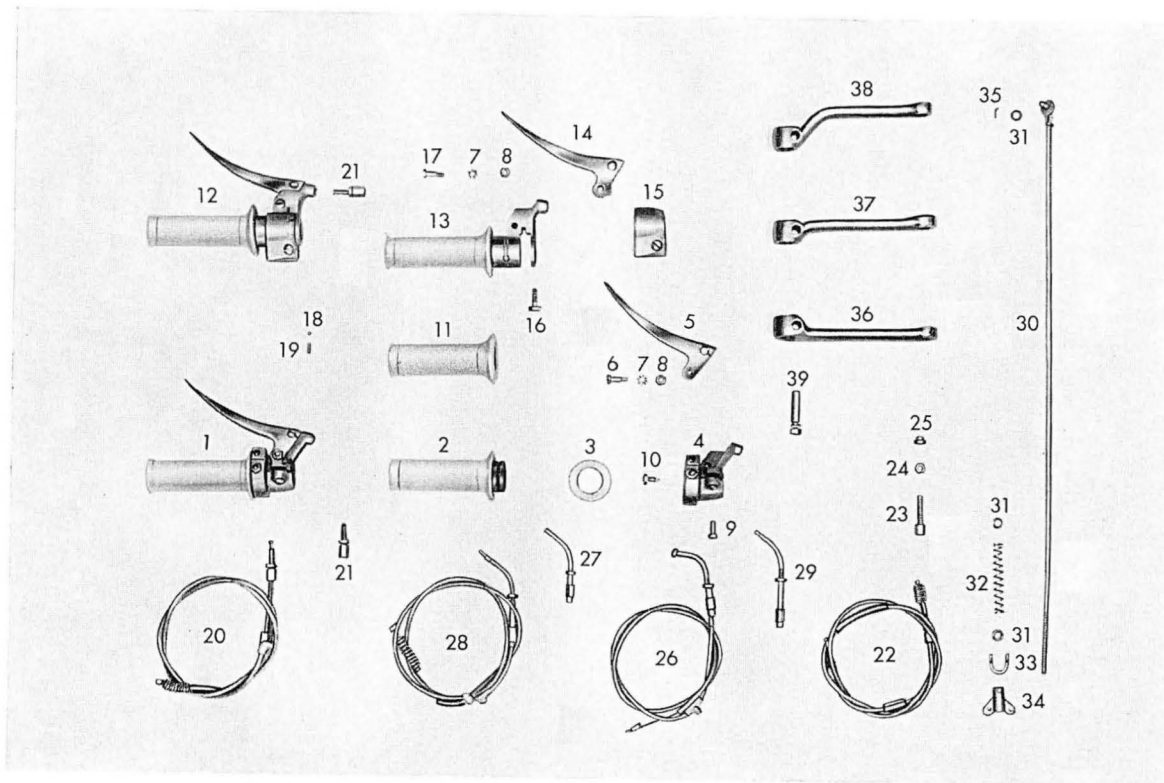
Tafel 8 Schalt-, Betätigungshebel-Züge
