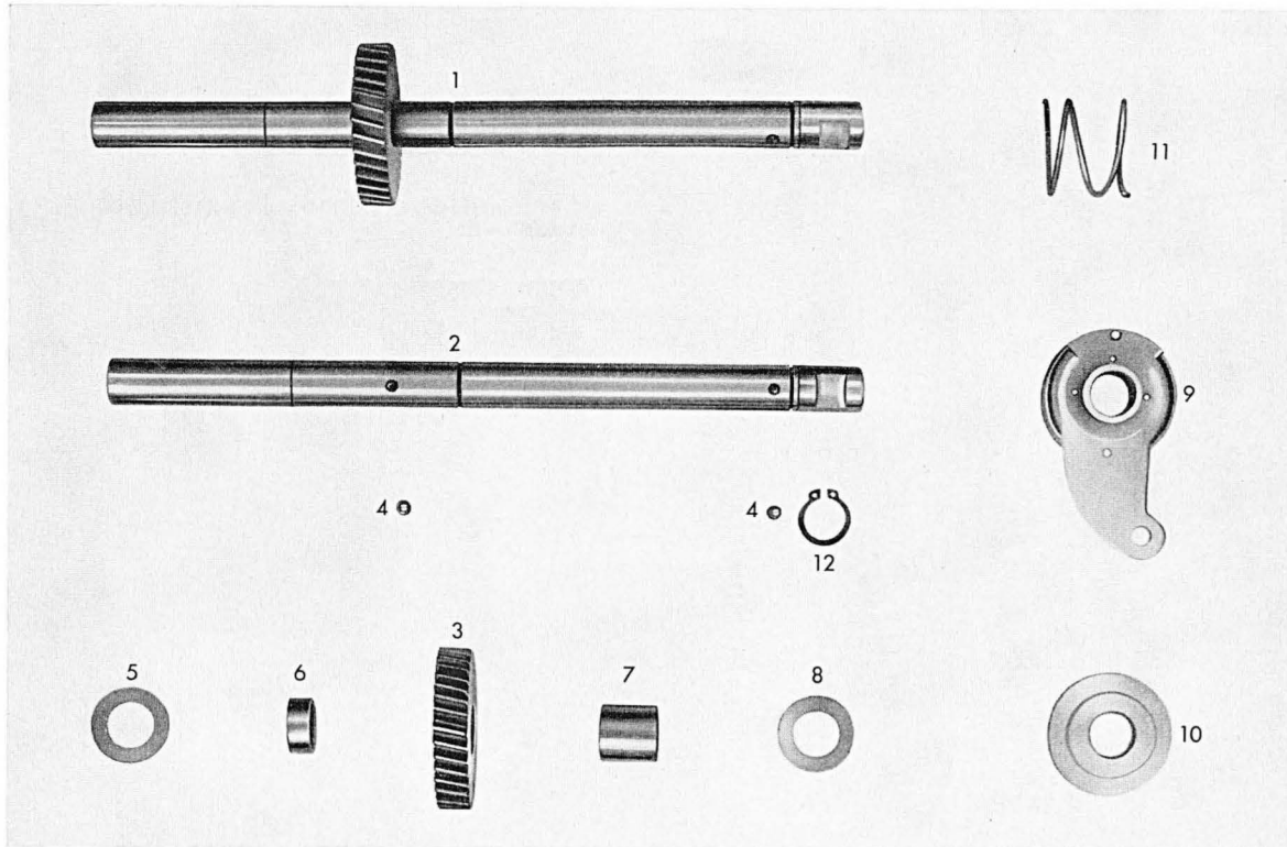
Tafel 9 Tretlagerachse - Bremshebel
