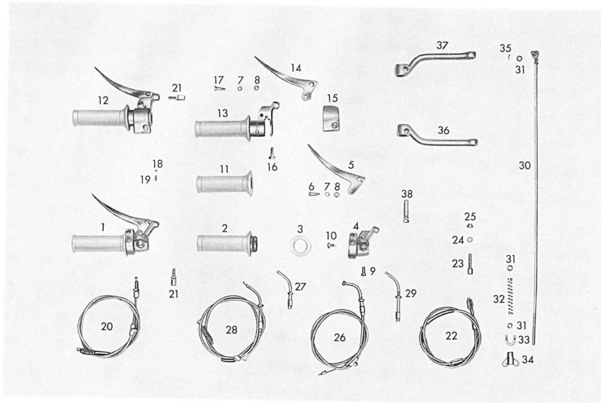
Tafel 8 a Schalt-, Betätigungshebel-Züge
