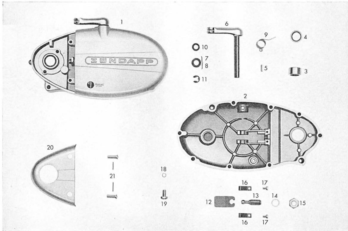
Tafel 4 a Gehäusedeckel rechts
