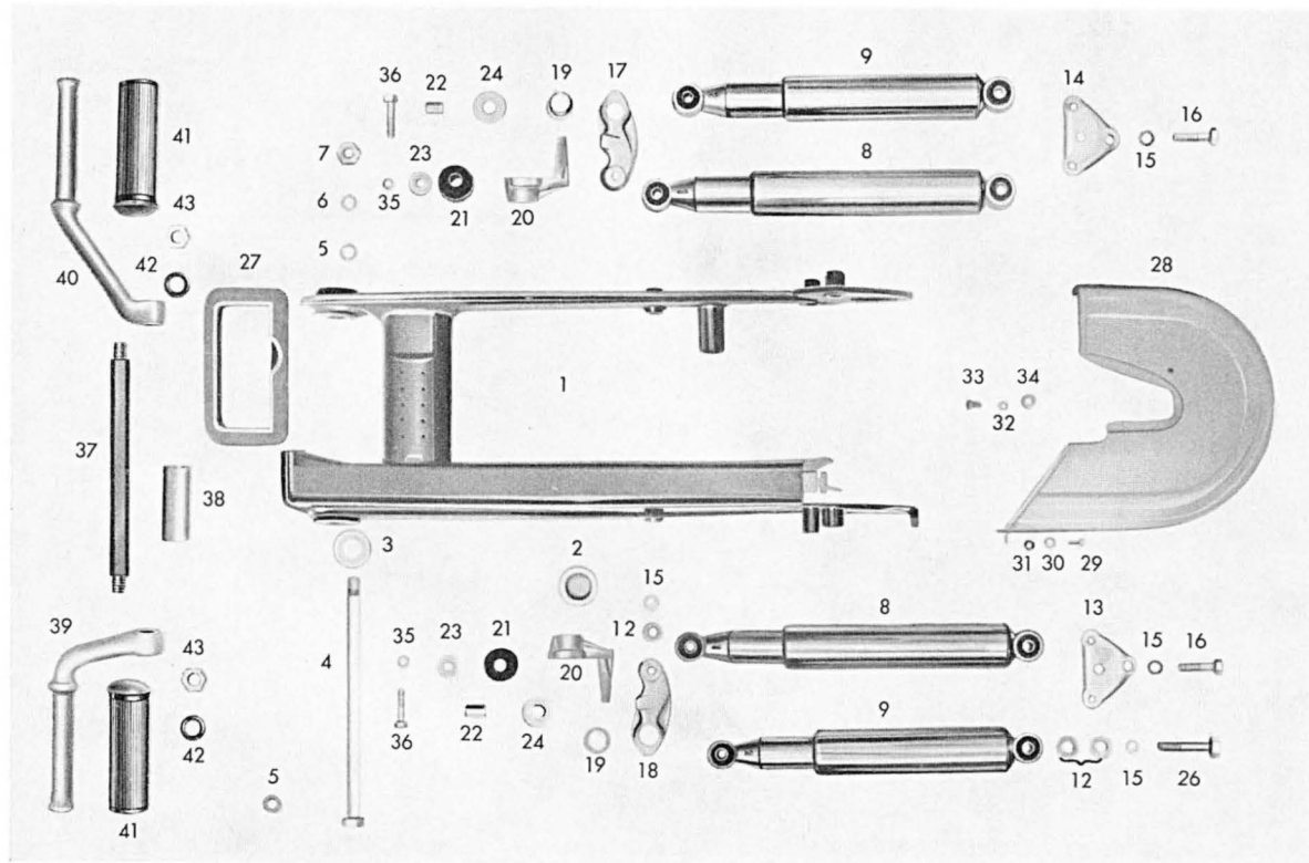
Tafel 4 a Hinterradgabel - Federbein - Fußrasten
