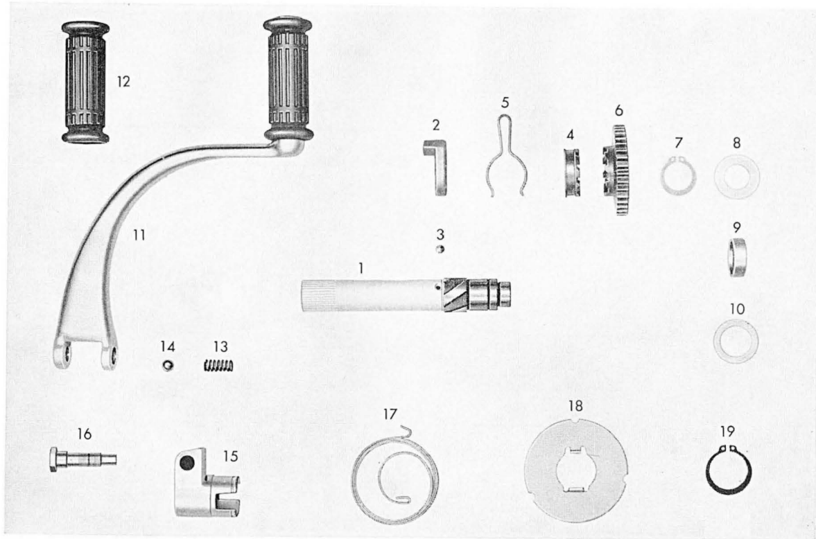
Tafel 9/1 Kickstarterwelle - Kickstarterhebel
