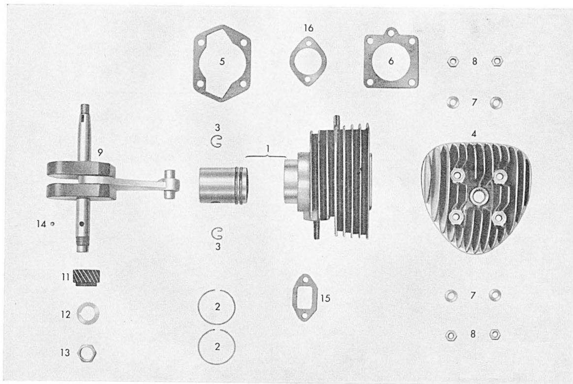
Tafel 5 a Zylinder - Kurbeltrieb (nur für Motoren ohne Gebläse)
