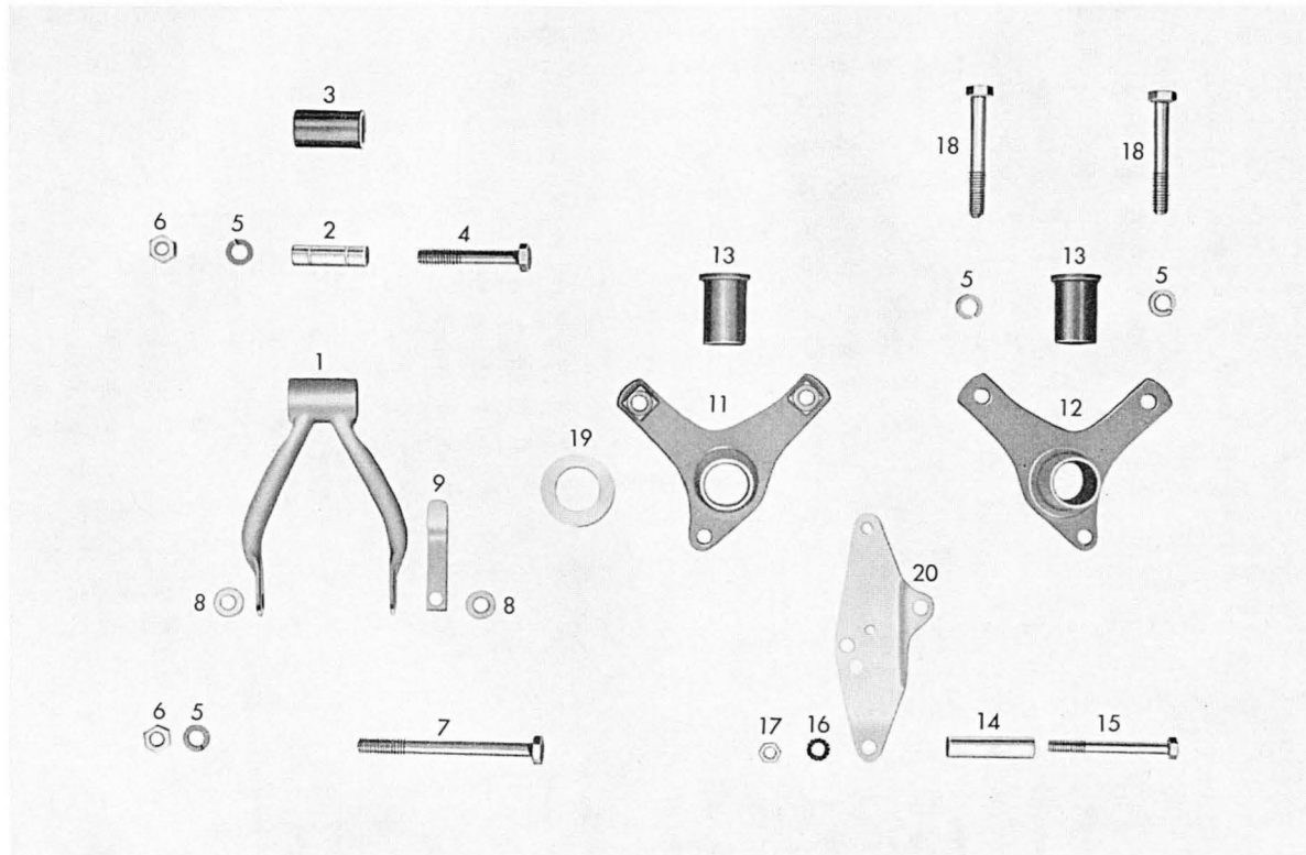
Tafel 2a Motoraufhängung
