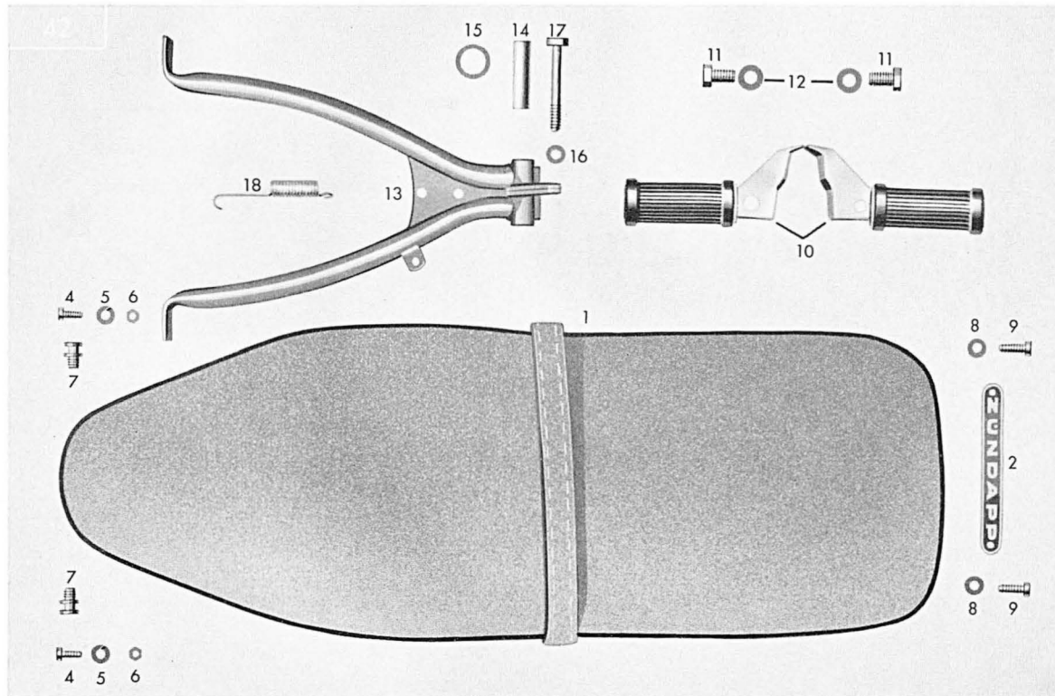
Tafel 12 a Doppelsitzbank - Einzelsitzbank - Radständer
