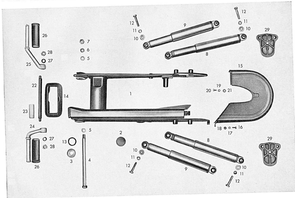
Tafel 4 b Hinterradgabel – Federbein, Fußrasten
