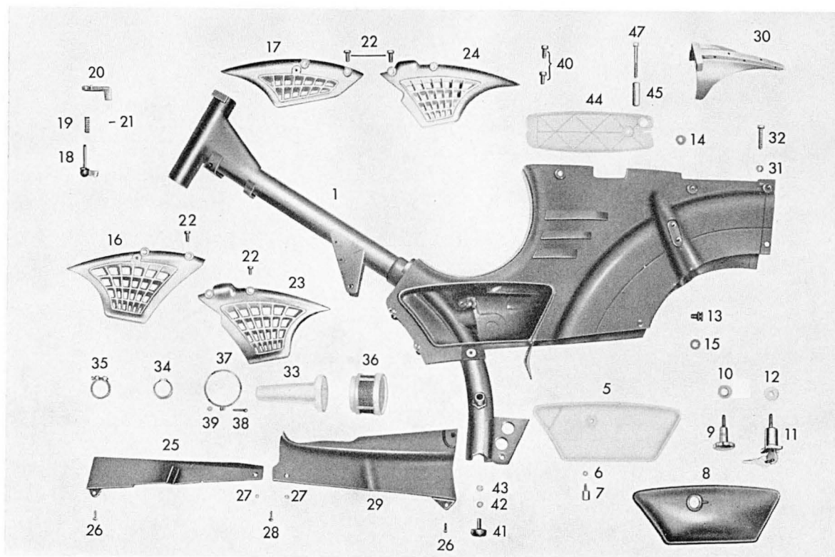
Tafel 1a Rahmen - Mittelteil
