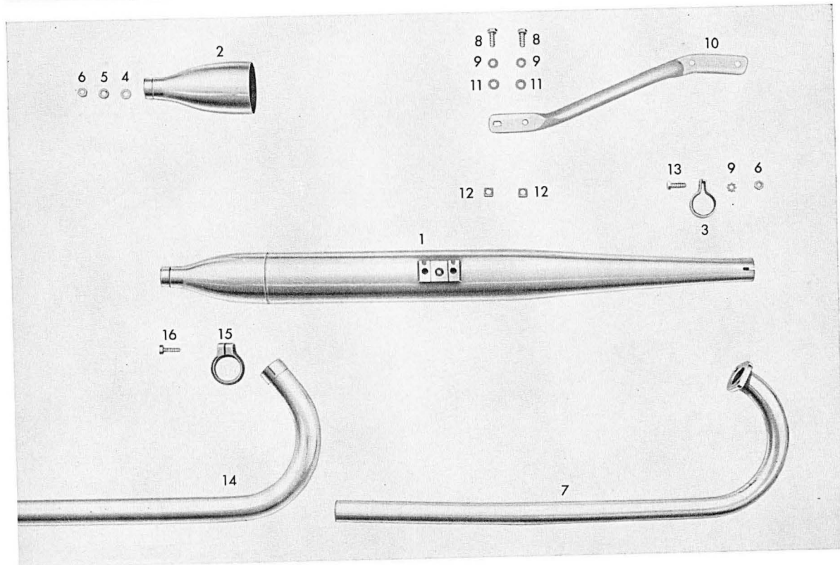
Tafel 12 b Auspuff
