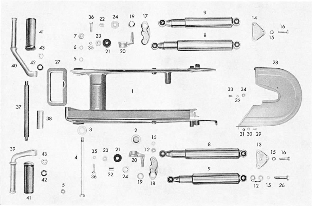
Tafel 4 a Hinterradgabel - Federbein - Fußbrasten
