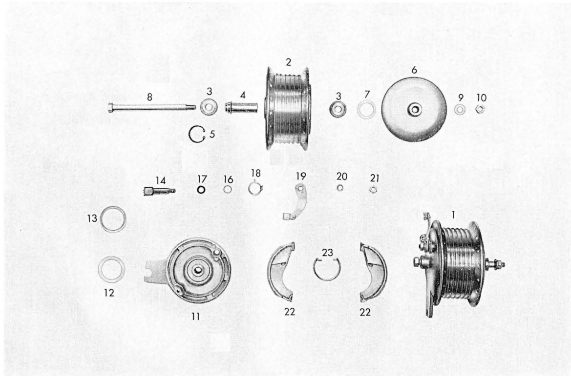
Tafel 5 Vorderes Laufrad - Vorderradnabe
