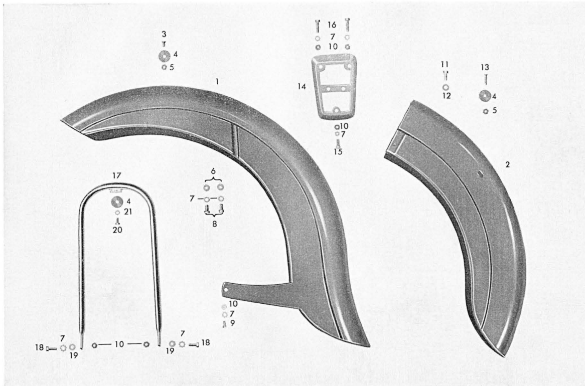
Tafel 9 a Schutzbleche
