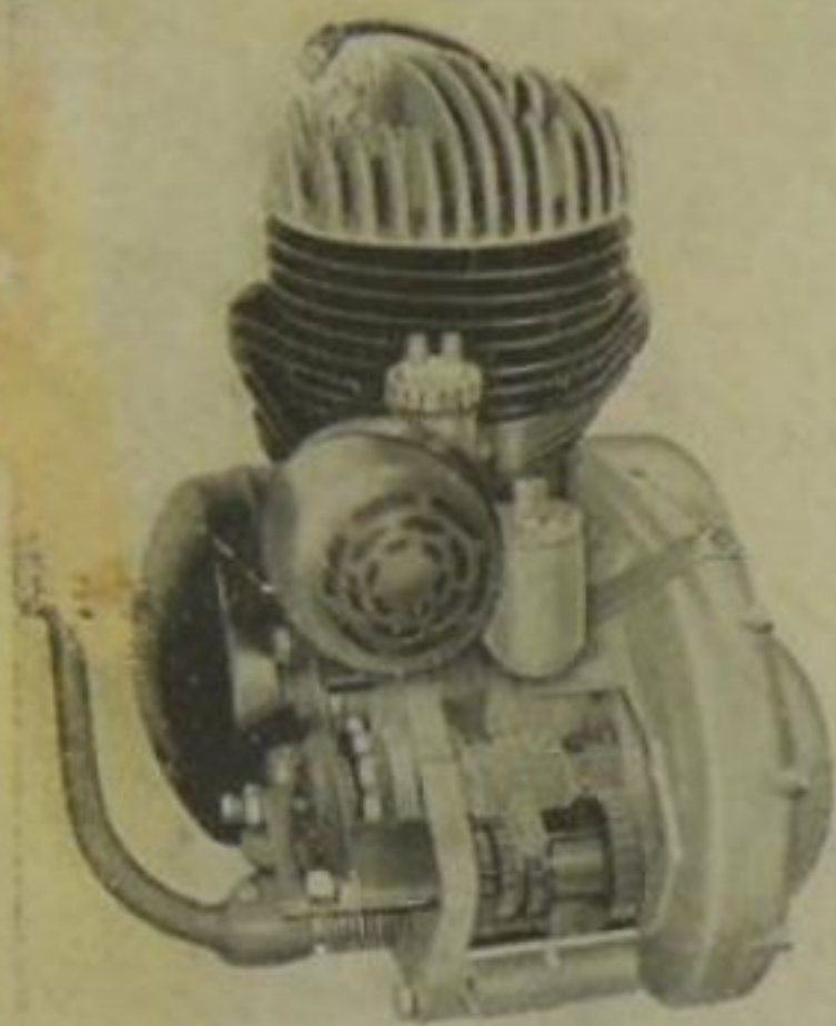
Motor mit Vierstrom-Spülung
