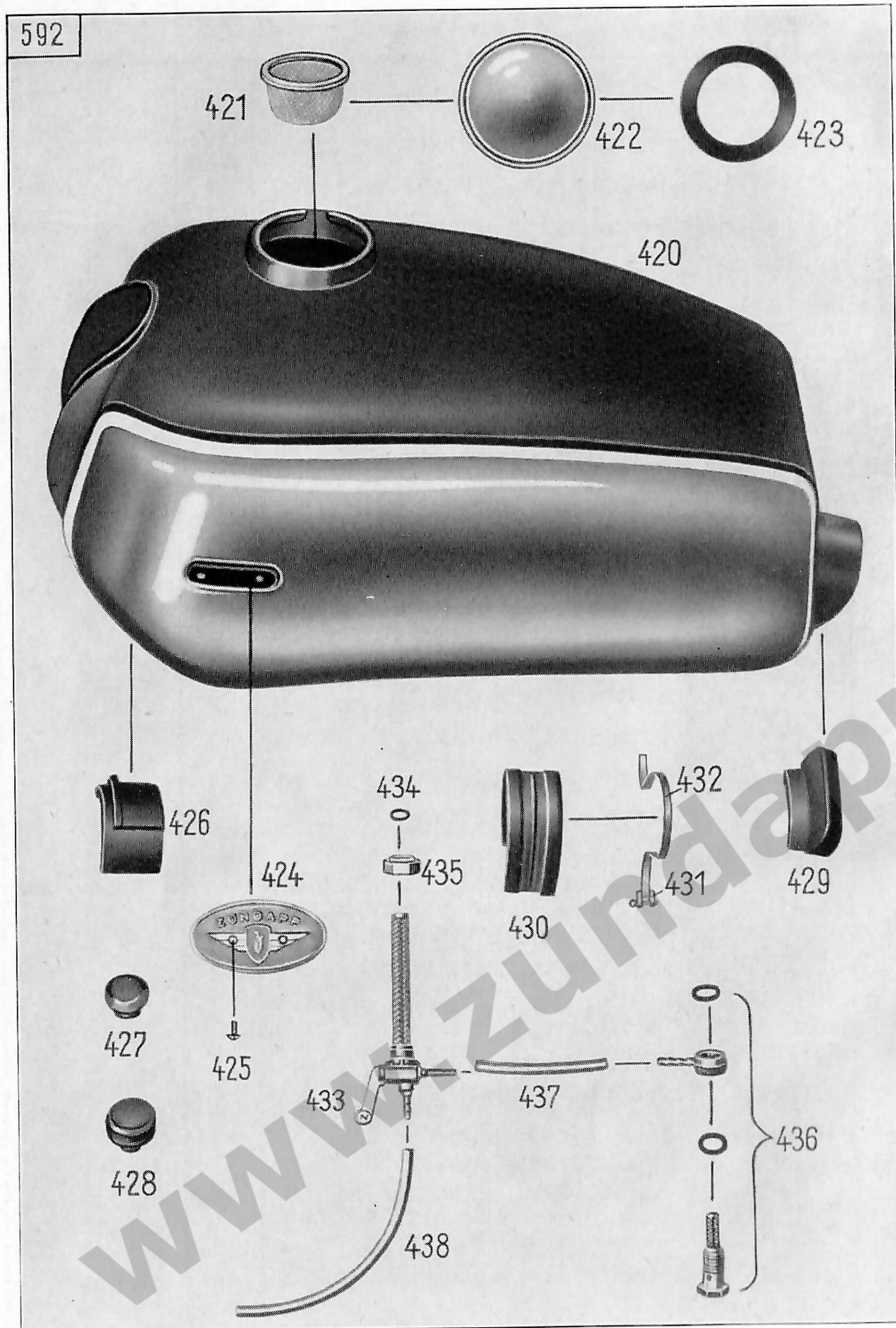
Tafel 17, Gruppe R: f) Kraftstoffbehälter und -leitungen
