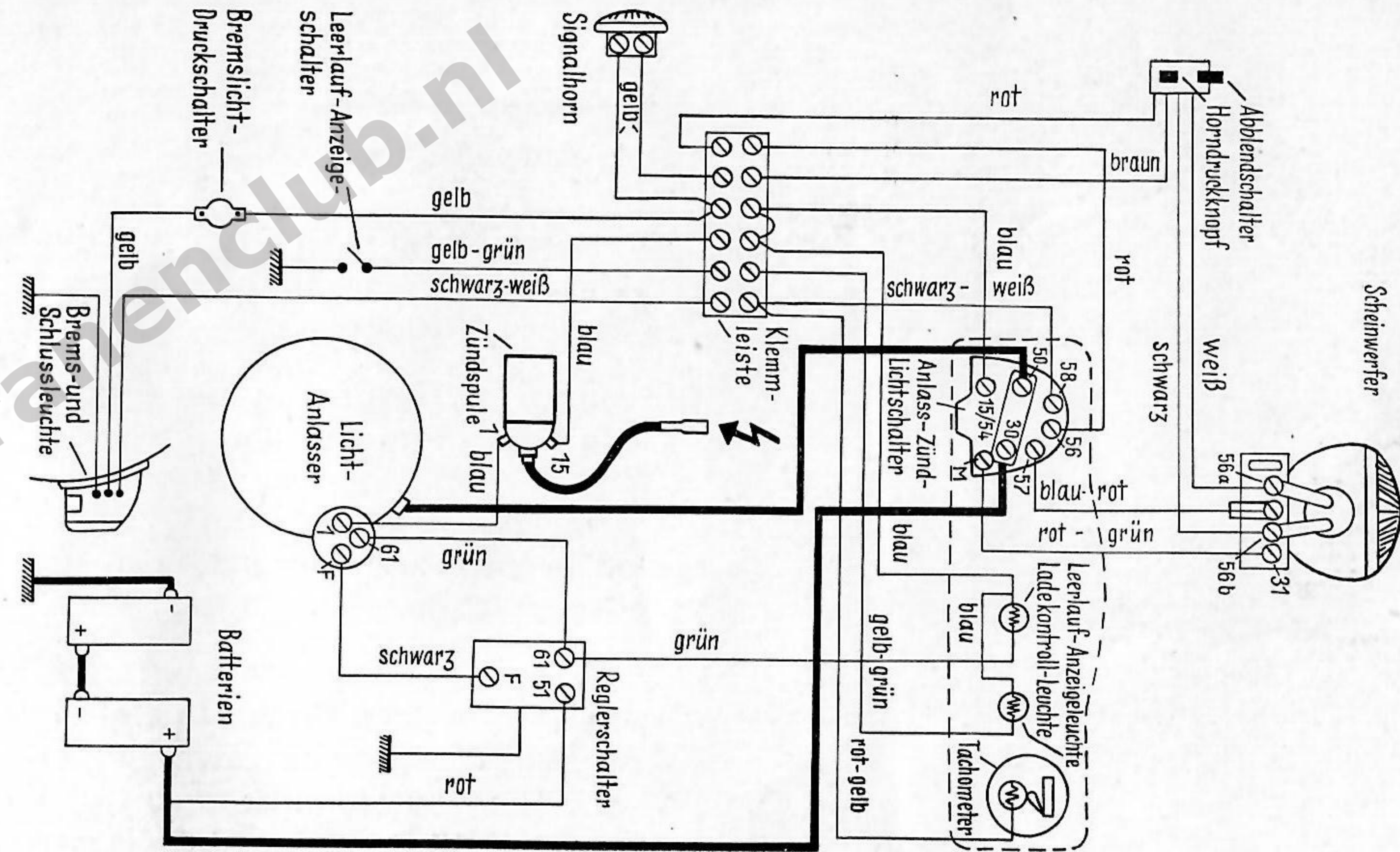
Schaltplan der elektrischen Anlage
