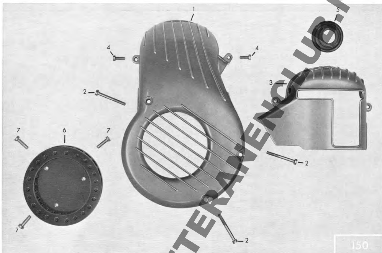
Tafel 3/1 Lüftergehäuse, Lüfterrad
