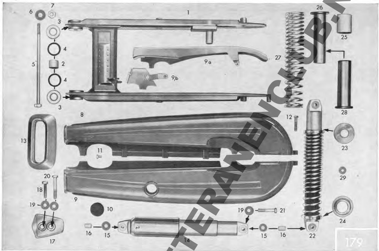
Tafel 28/1 Hinterradgabel, Federbein, Kettenschutz
