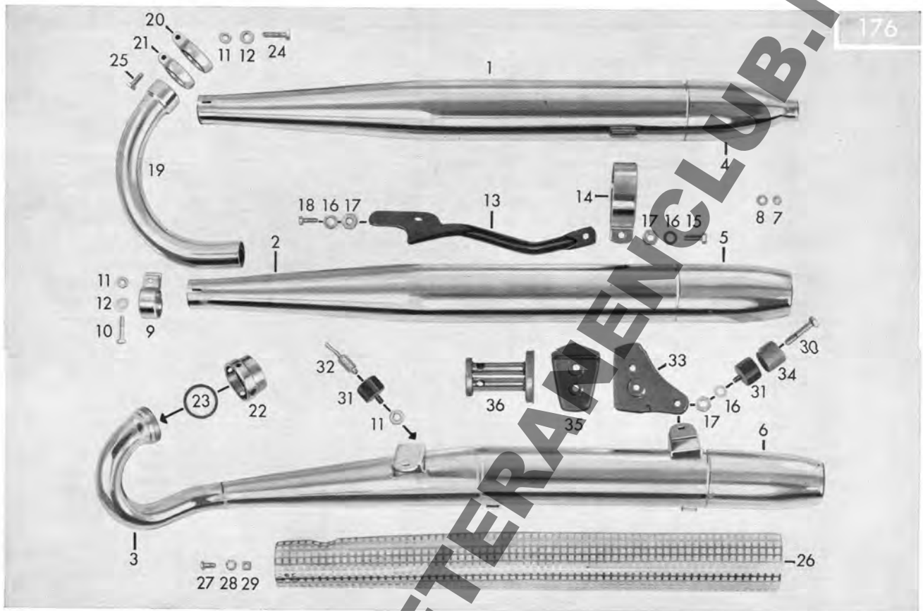
Tafel 24/2 Auspuff-Anlage
