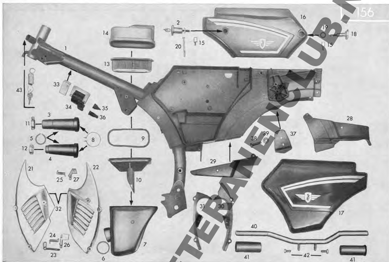
Tafel 25/3 Rahmen, Ansauggeräuschdämpfer, Vergaserverkleidung, Fußrastenrohr
