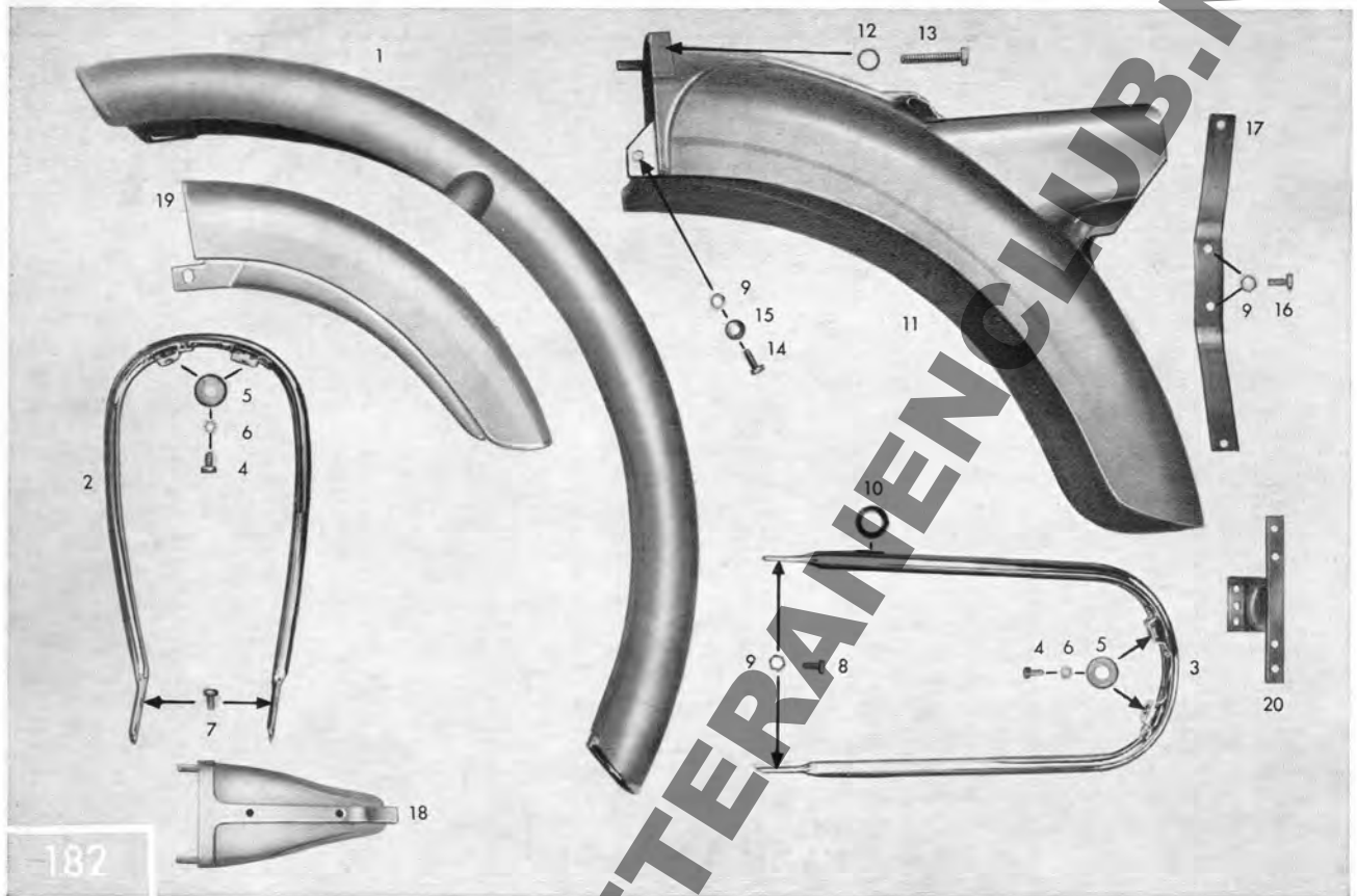
Tafel 36/1 Schutzbleche, Zierbügel, Nummernschildhalter
