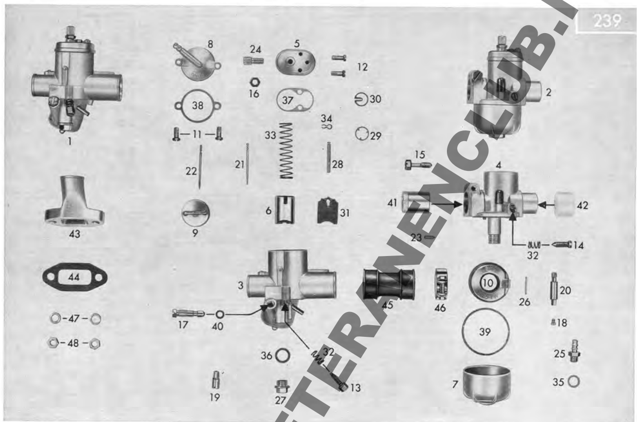
Tafel 6/3 Vergaser, Ansaugung
