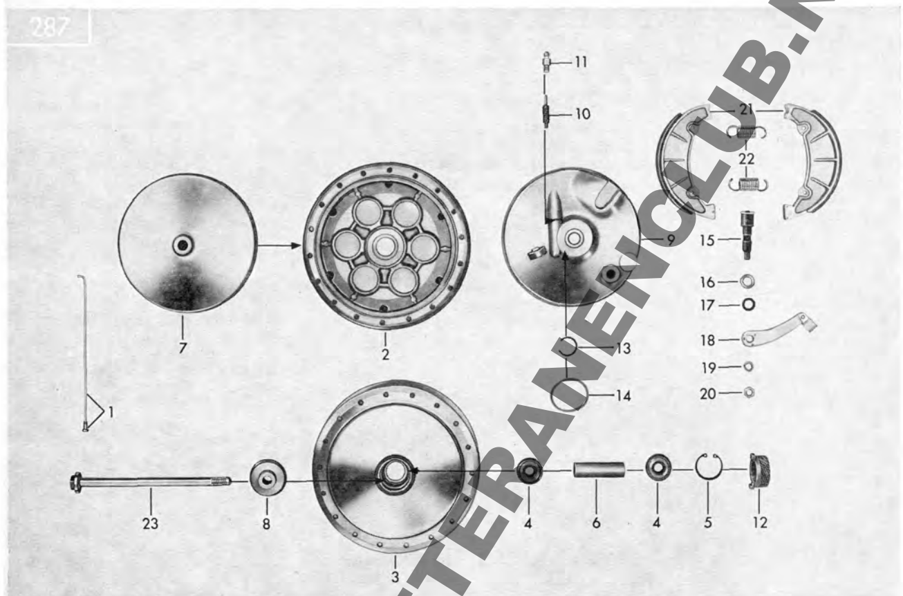
Tafel 30/2 Vorderes Laufrad, Vorderradnabe 150 mm \phi
