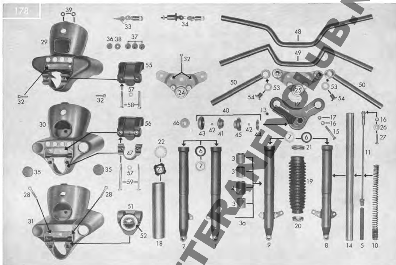
Tafel 27/1 Vorderradgabel, Gabelgehäuse, Lenkungslager, Lenker
